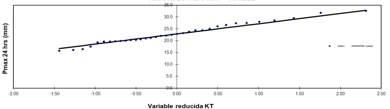
AJUSTE ESTADISTICO - GUMBEL
