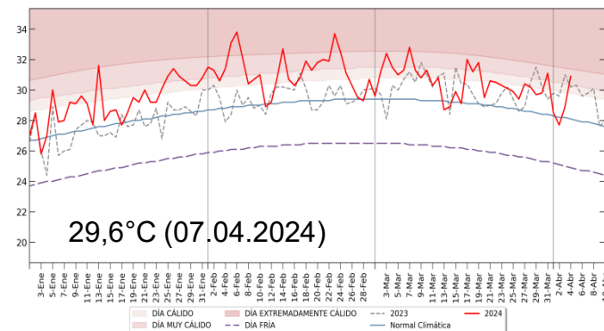
TEMPERATURA MÁXIMA [°C] ESTACIÓN: VON HUMBOLDT - LIMA
