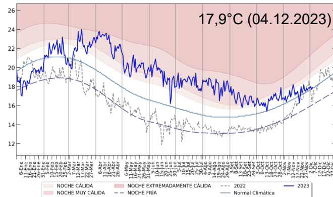
TEMPERATURA MÍNIMA [°C] ESTACIÓN: CAMPO DE MARTE - LIMA
