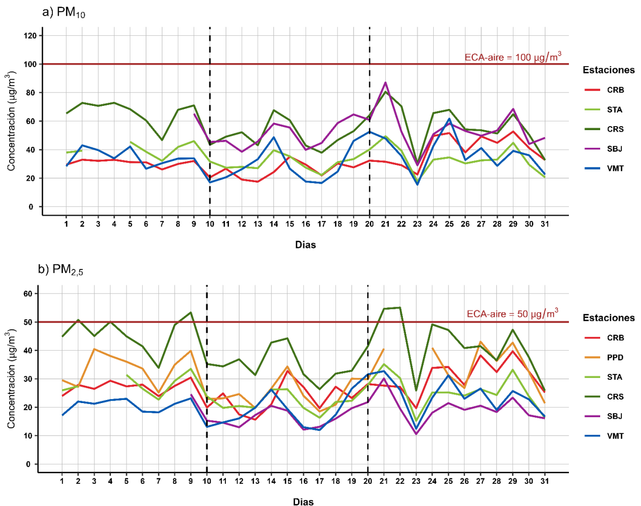
Figura N°07. Variación diaria del PM 10 y PM 2.5 (µg/m 3 ) en el AMLC.
