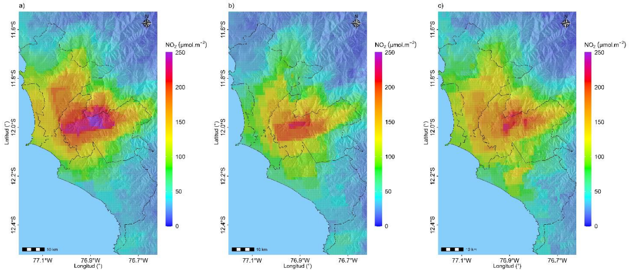
Figura N°09. Distribución espacial de la columna del NO 2 (μmol/m 2 ) en la troposfera del AMLC.
