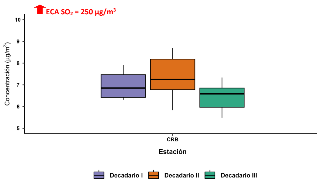
Figura N° 14. Variación horaria del SO 2 (µg/m 3 ) en el AMLC.
