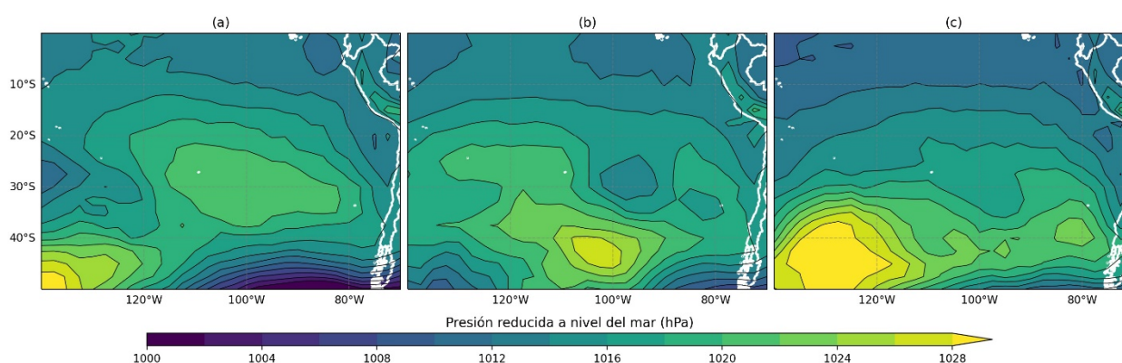
Figura N°01. Promedio decadiario de la presión atmosférica (hPa) a nivel del mar.
