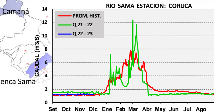
Figura 4 Caudales diarios de los ríos de la zona sur de la RHP
