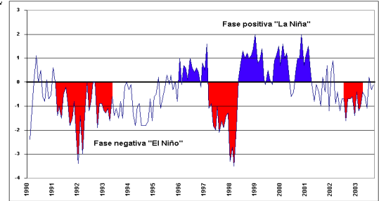
Figura 5. Índice de Radiación de Onda Larga
