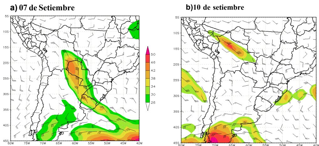
Figura 10. Isotacas (LLJ/SJ mayores de 25 Nudos
