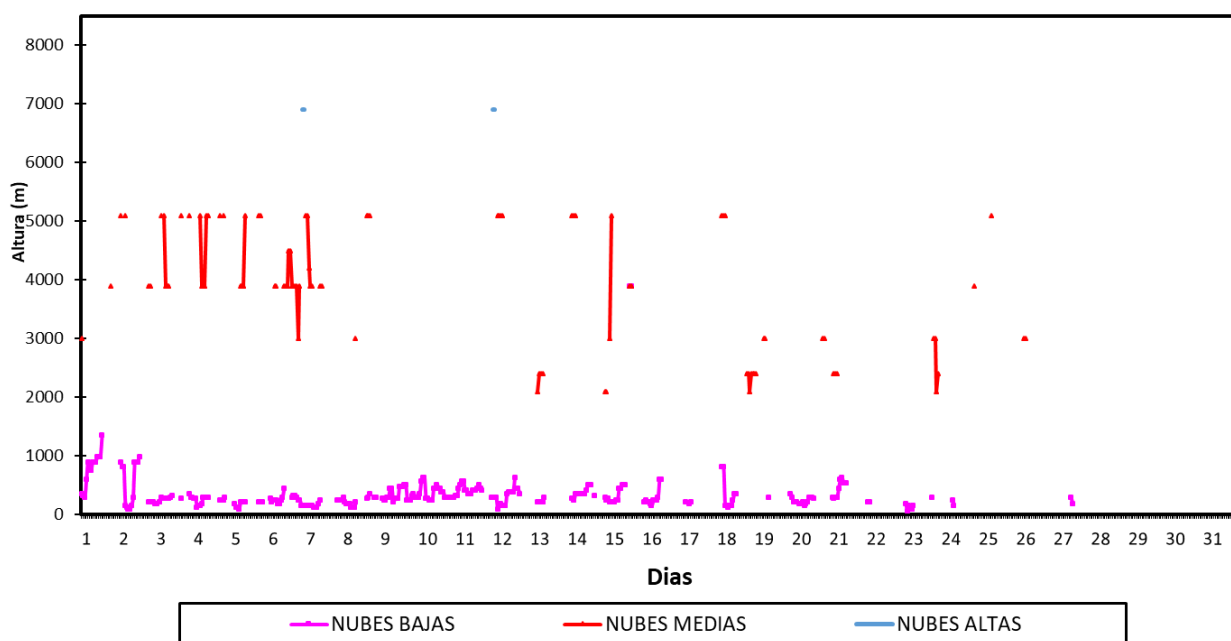
Figura N° 05. Altura de la base de nube (m) registrada en la estación Aeropuerto Internacional Jorge Chávez (JCH).
