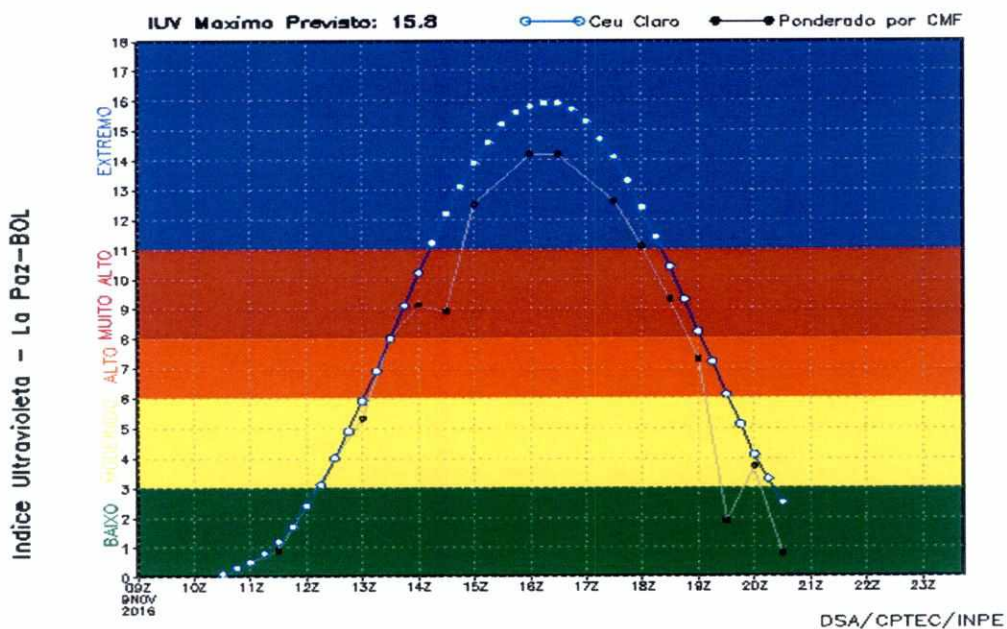
Figura 22: Pronóstico de UVI máximo para La Paz Bolivia para el 9/11/2016 (CPTEC) 57
