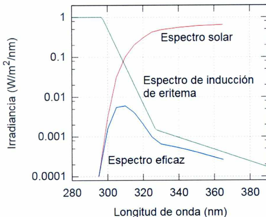
Figura 3: Irradiancia espectral UV y el espectro de acción eritemática 18
