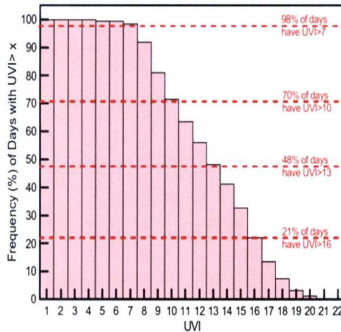
Figura 20: Distribución acumulada de UVI máximo para La Paz Bolivia para el período 2008 – 2012)
