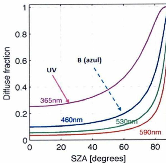
Figura 7: Difusión (en función de longitud de onda) vs Ángulo Cenital Solar (SAZ)
