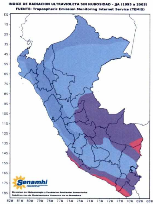
Figura 18: UVI potencial para el invierno (cielo despejado)
