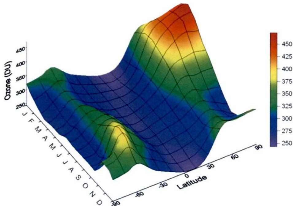
Figura 13: Ozono total mensual (DU) en función de la latitud (período 1964–1980)
