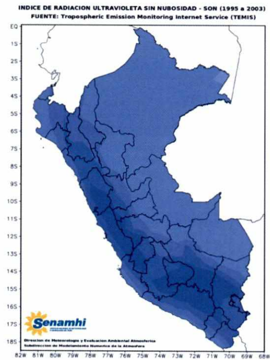
Figura 19: UVI potencial para la primavera (cielo despejado)
