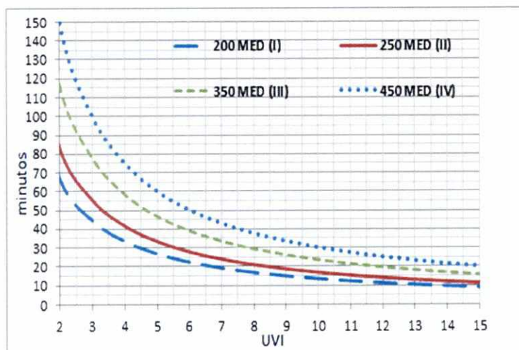
Figura 23: Tiempo de exposición en minutos asociado a MED según tipo de piel
