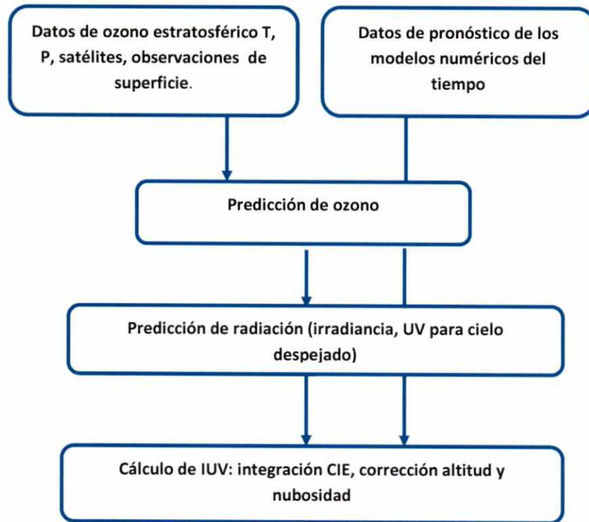
Figura 12: Esquema del proceso de pronóstico de UVI 43
