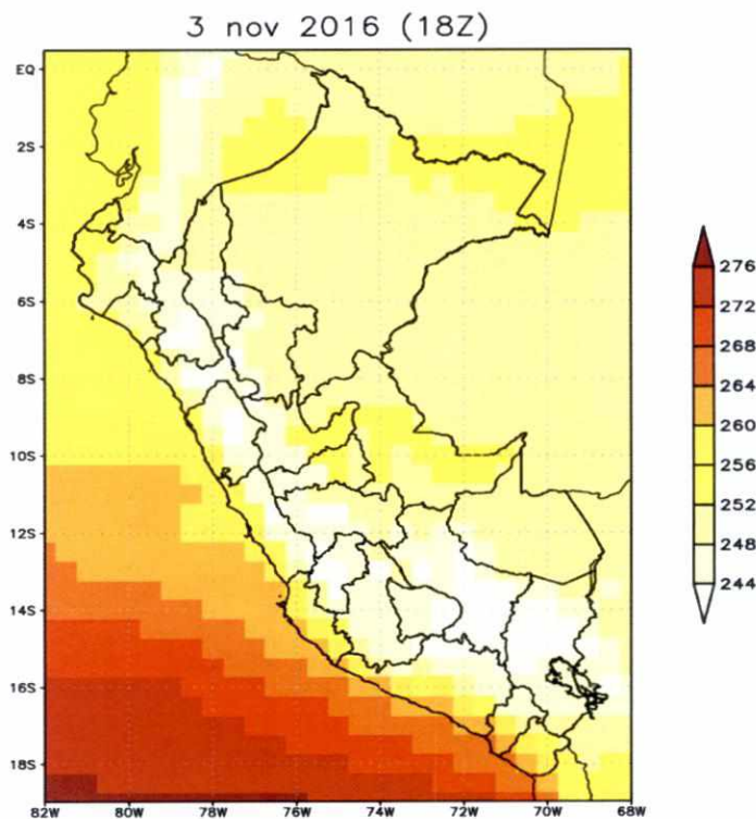
Figura 15a: Pronóstico de columna de ozono en UD para la 1 pm (GFS NOAA)
