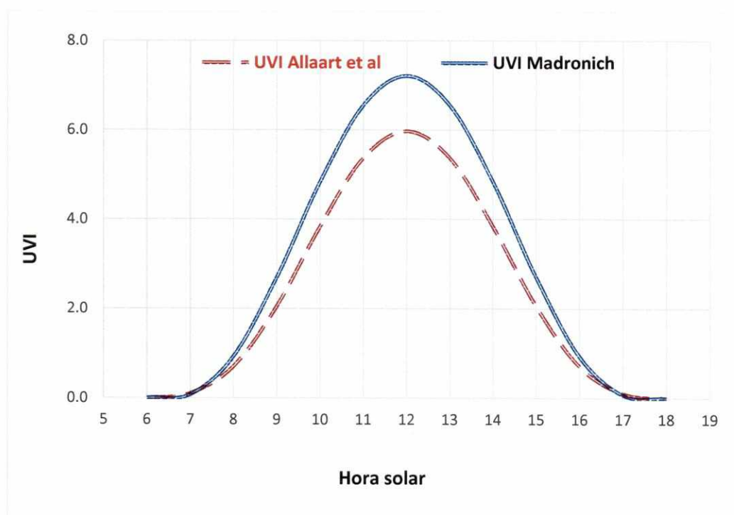
Figura 10: Estimación de UVI usando las fórmulas Allaart, Madronich para el 21 Junio de 2016
