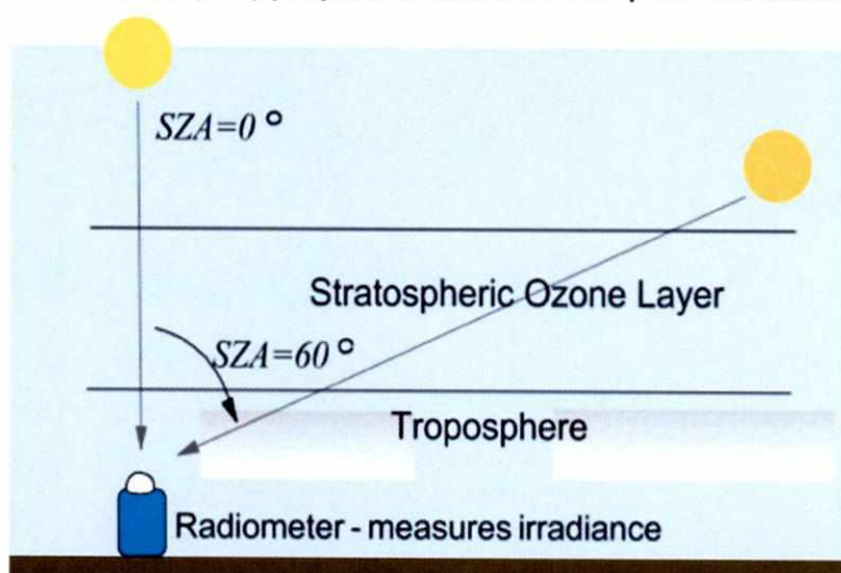
Figura 5: El ángulo cenital solar (SZA) y capa de ozono son claves para la estimación del UVI
