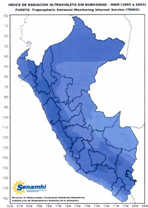
Figura 17: UVI potencial para el otoño (cielo despejado)
