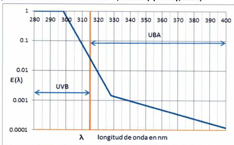
Figura 2: Espectro de acción eritemática 12 (McKinlay y Diffey, 1987)
