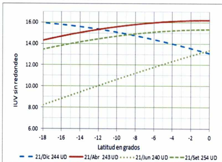
Figura 14: Variación del UVI según latitud considerando valores típicos de ozono (período 2000 – 2015) en la Estación VAG - Marcapomacocha
