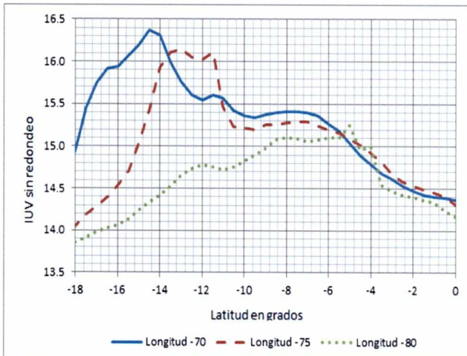
Figura 15b: Pronóstico para cielo despejado de UVI para la 1 pm del 3/11/2016 (NOAA), corte longitudinal
