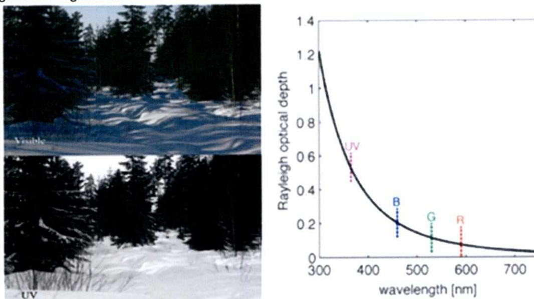
Figura 6: Fotografía banda visible vs banda UV
