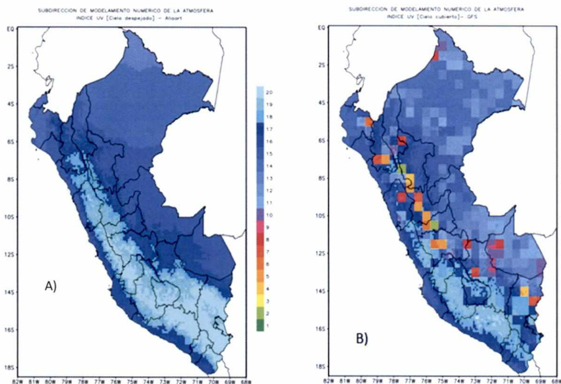
Figura 24: Pronóstico del Índice UV máximo para el día 4 de diciembre
