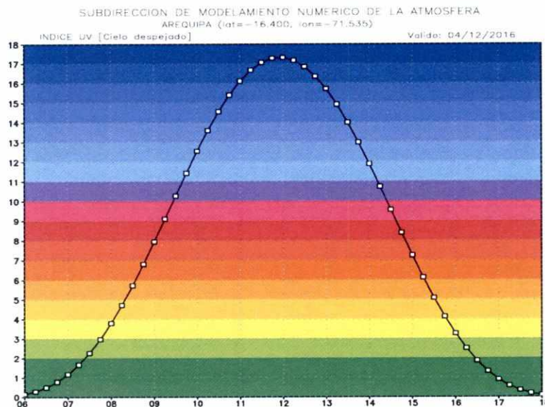
Figura 25: Pronóstico del Índice UV horario para la ciudad de Arequipa, para el 4 de diciembre. La línea negra es el pronóstico para cielo despejado mediante la parametrización de Allaart
