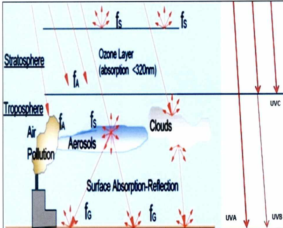
Figura 11: Los modelos de transferencia radiativa deben tomar en cuenta la interacción entre la radiación entrante y nuestra atmósfera
