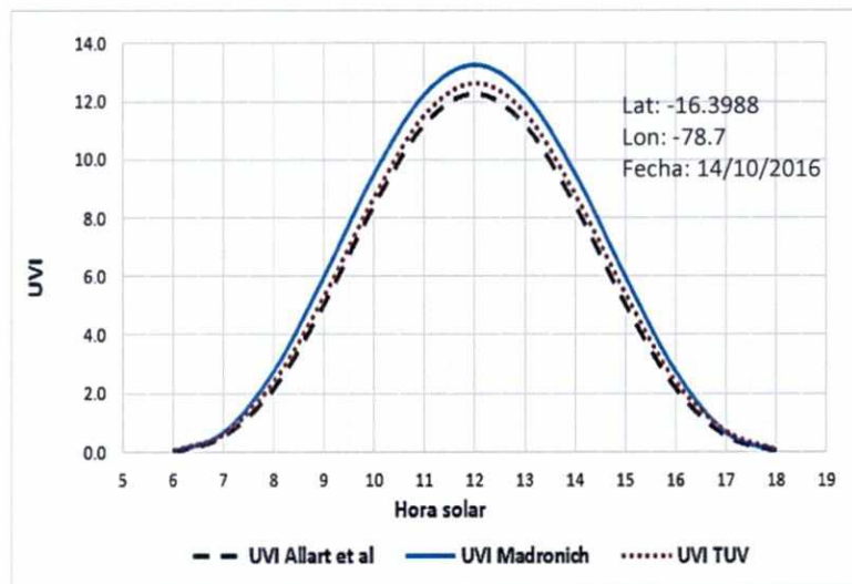
Figura 9: Estimación de UVI usando las fórmulas Allaart, Madronich y el modelo TUV
