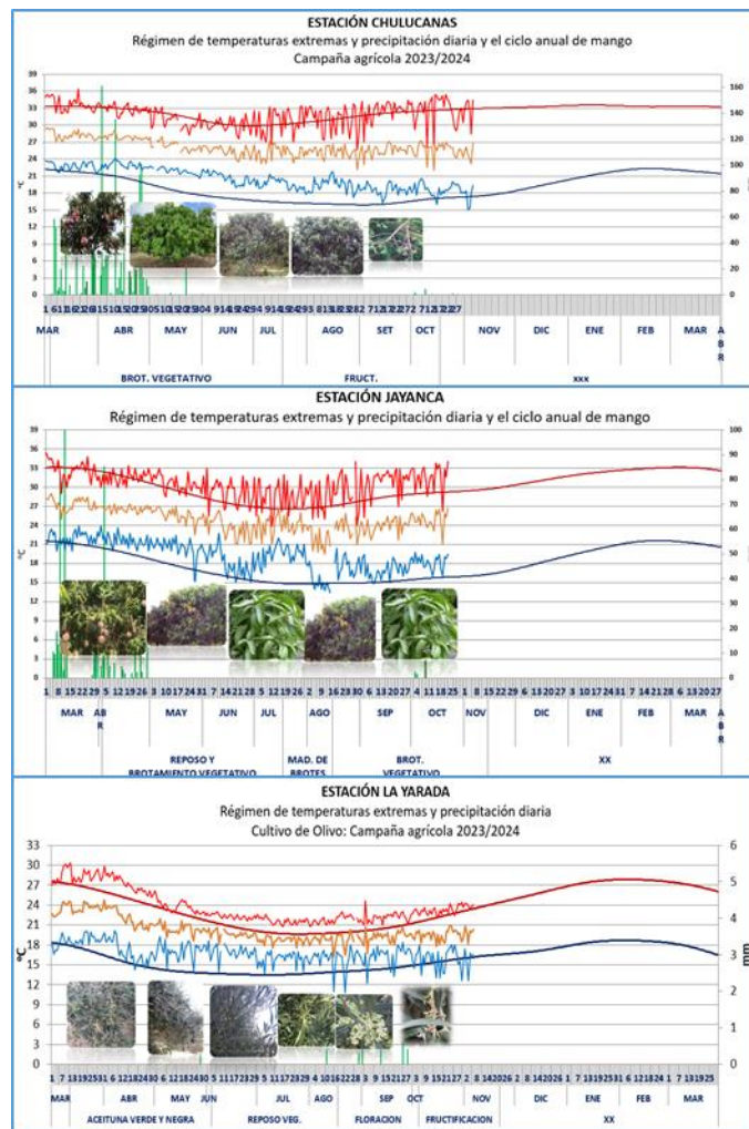
Figura 40. Monitoreo agrometeorológico del mango y olivo campañas agrícolas 2023/2024 en las estaciones de Jayanca, Chulucanas y La Yarada. Fuente: SENAMHI
