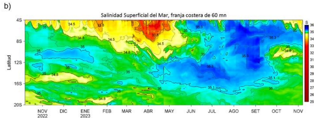
Figura 26. (a) Distribución quincenal de la Salinidad Superficial del Mar (SSM) en el Pacífico Sudeste, durante el mes de 7 de setiembre y 9 de octubre del 2023. (b) Diagrama Hovmöller de la SSM en la franja de las 60 millas costeras, al 7 de noviembre de 2023. Datos:
