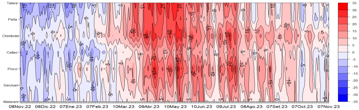
Figura 18. Evolución diaria de las anomalías del nivel del mar en el litoral de Perú del 08 de noviembre 2022 al 07 de noviembre 2023, Climatología: 1991-2020. Procesamiento: DIHIDRONAV.
