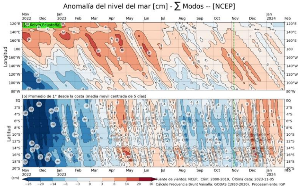
Figura 37. Igual que la Figura 41 pero el modelo es forzado con los vientos del reanalysis de NCEP. Fuente: IGP.
