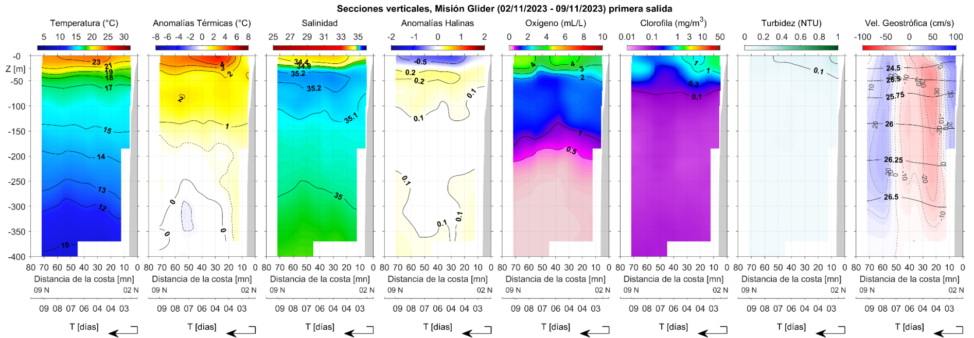
Figura 21. Secciones verticales de temperatura (°C), anomalías térmicas (°C), salinidad, anomalías halinas, oxígeno (mL L -1 ), clorofila (mg m -3 ), turbidez (NTU) y corrientes geostróficas (cm s -1 ), a partir de los datos registrados por el glider Mochica frente a Negritos – Talara (entrada y salida), registrados desde el 02 de noviembre hasta el 9 de noviembre.
