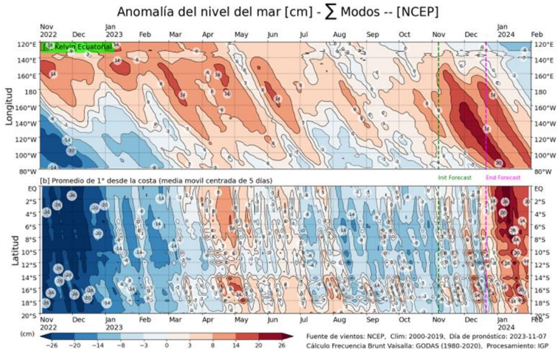
Figura 38. Igual que la Figura 42, pero para el pronóstico de los siguientes 41 días (entre la línea vertical verde y rosada) se usa la información de anomalías de vientos del modelo atmosférico CFSv2. Luego de la línea rosada, los vientos usados para el pronóstico fueron iguales a cero. Fuente: IGP denominada NCEP. Fuente: IGP
