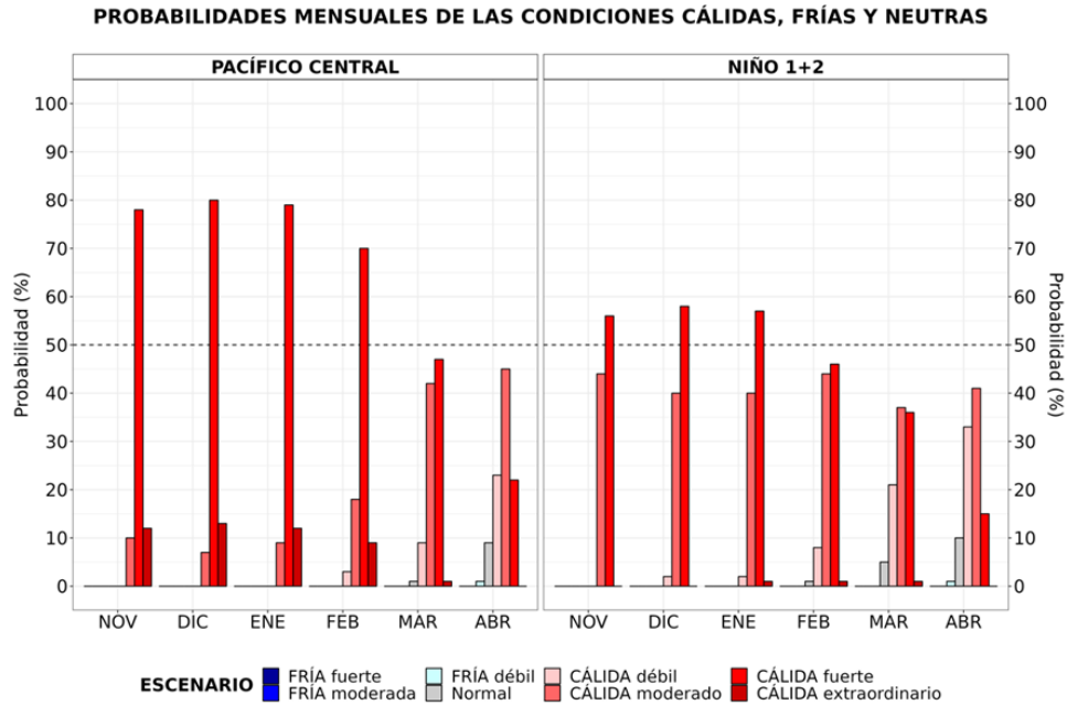
Figura 39. Probabilidades mensuales estimadas para condiciones cálidas, neutras y frías en el Pacífico central (región Niño 3.4, izquierda) y en el extremo del Pacífico oriental (región Niño 1+2, frente a la costa de Perú, derecha) entre noviembre y abril 2024.
