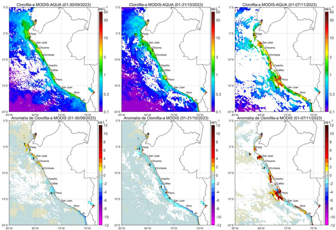
Figura 29. Distribución de la concentración de clorofila-a superficial satelital ( \mu\text{g L}^{-1} , panel superior) y su anomalía ( \mu\text{g L}^{-1} , panel inferior), durante agosto, setiembre y lo que va de noviembre de 2023 (de izquierda a derecha), proveniente de MODIS-AQUA. Fuente: Fuente: Satélite MODIS. Procesamiento: LHQ/AFIOQG/DGIOCC/IMARPE.
