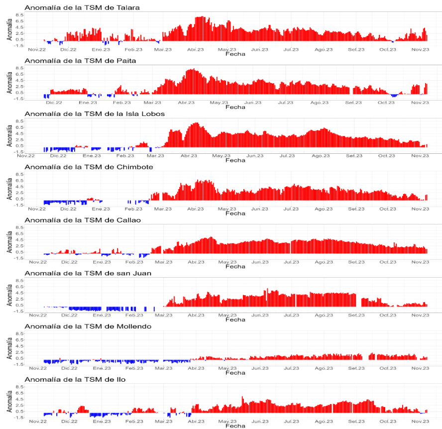
Figura 115. Anomalia de la TSM diaria a lo largo del litoral de Perú de noviembre 2022 a noviembre 2023. Climatología: 1991-2020. Fuente: DIHIDRONAV.
