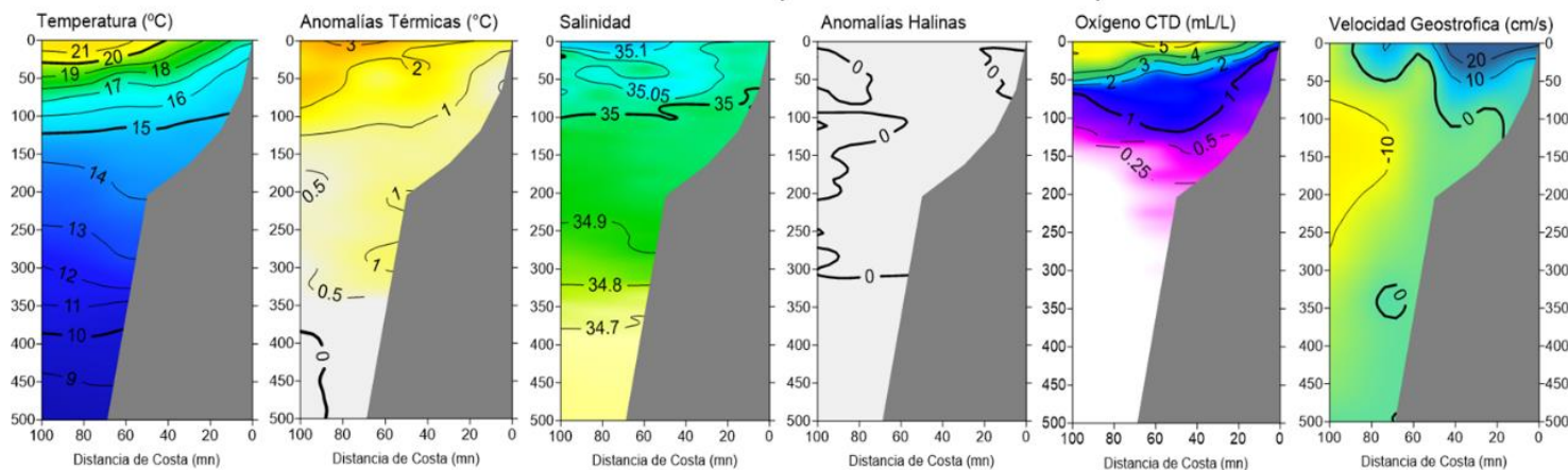
Figura 23. Secciones oceanográficas de temperatura, anomalía térmica, salinidad, anomalía halina, y oxígeno disuelto, realizadas frente a Paíta y Chicama, dentro de las 100 mn, entre el 21 y 24 de octubre de 2023. Climatología: 1991-2020 (Domínguez et al., 2023).
