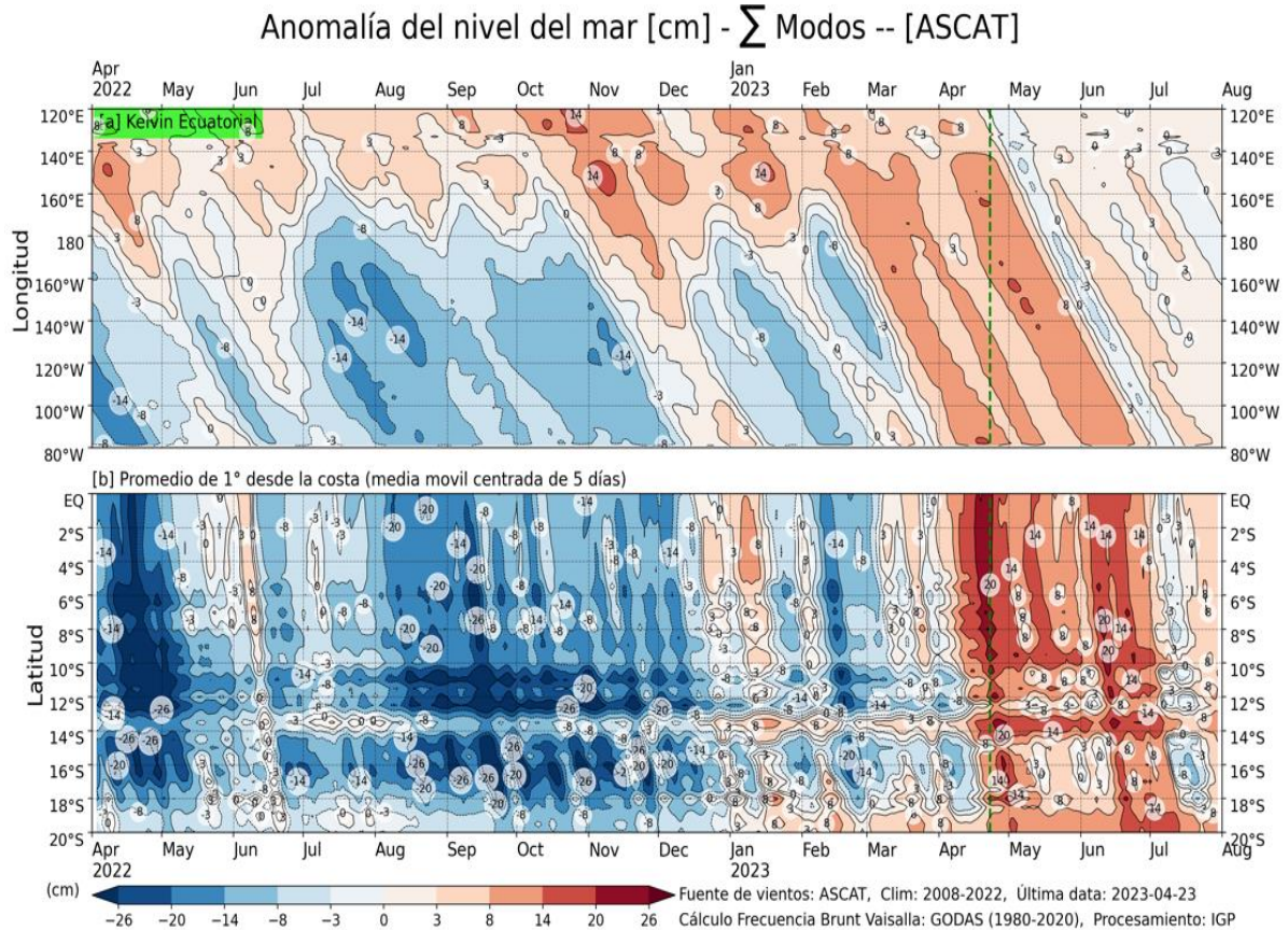
Figura 32. Anomalía del nivel del mar (en cm) para la sumatoria de los modos (modo 1, 2 y 3) simulado a partir del Modelo Oceánico Multimodal (MOMM-IGP; Urbina y Mosquera, 2020) en la franja ecuatorial (superior) y costera (inferior), La línea verde representa el inicio del pronóstico, el modelo fue forzado con la fuente de datos de viento denominada ASCAT.
