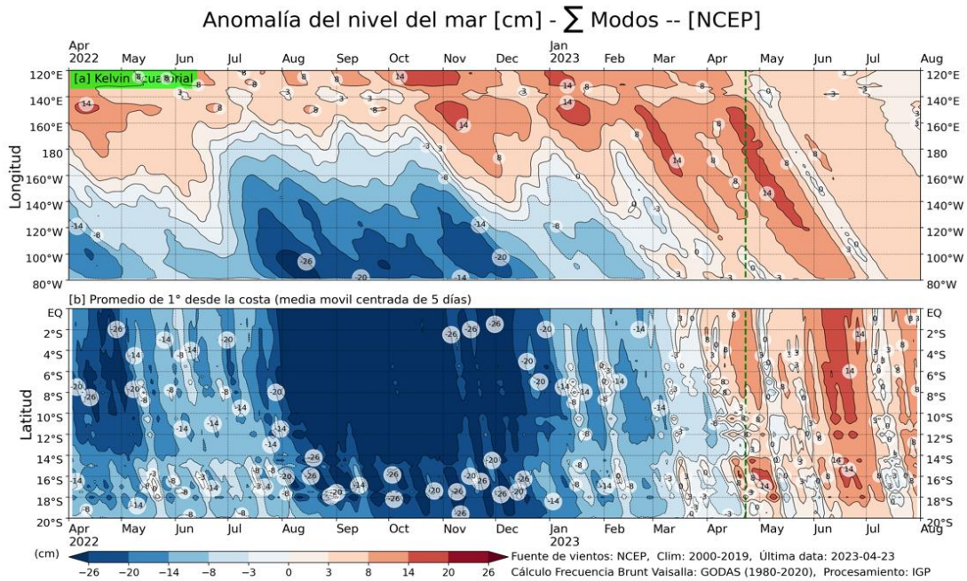
Figura 33. Anomalía del nivel del mar (en cm) para la sumatoria de los modos (modo 1, 2 y 3) simulado a partir del Modelo Oceánico Multimodal (MOMM-IGP; Urbina y Mosquera, 2020) en la franja ecuatorial (superior) y costera (inferior), La línea verde representa el inicio del pronóstico, el modelo fue forzado con la fuente de datos de viento denominada NCEP.
