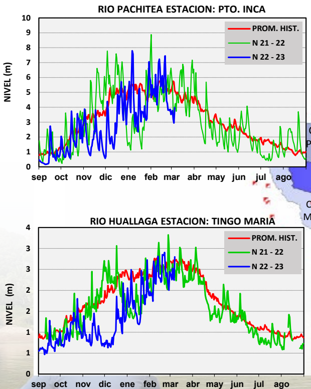
Figura 10 Caudales y niveles diarios de los ríos de la RHA zona centro y sur.
