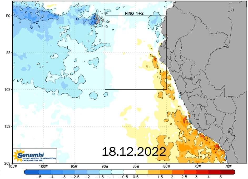
SENAMHI/DMA/SPM OSTIA - ANOMALIA DE LA TEMPERATURA SUPERFICIAL DEL MAR (°C) 18 de Diciembre de 2022
