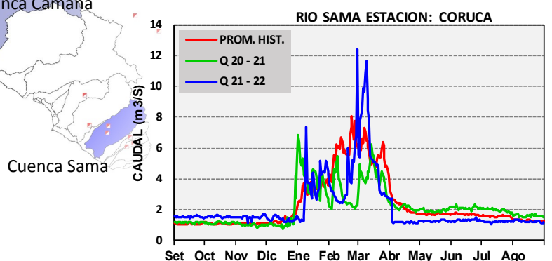
Figura 4 Caudales diarios de los ríos de la zona sur de la RHP
