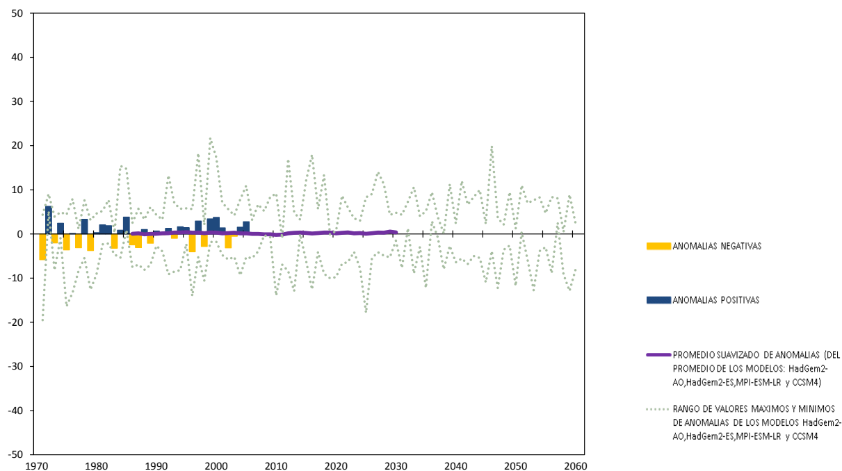
Figura 6. Evolución del cambio de la precipitación en las subgrillas (ajustadas con datos observados del CRU 3 ), expresado en porcentaje (%).
