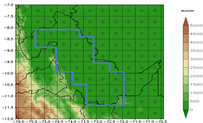
Figura 5. Subgrillas analizadas para determinar la tendencia de cambio en la región Ucayali. Fuente SENAMHI.
