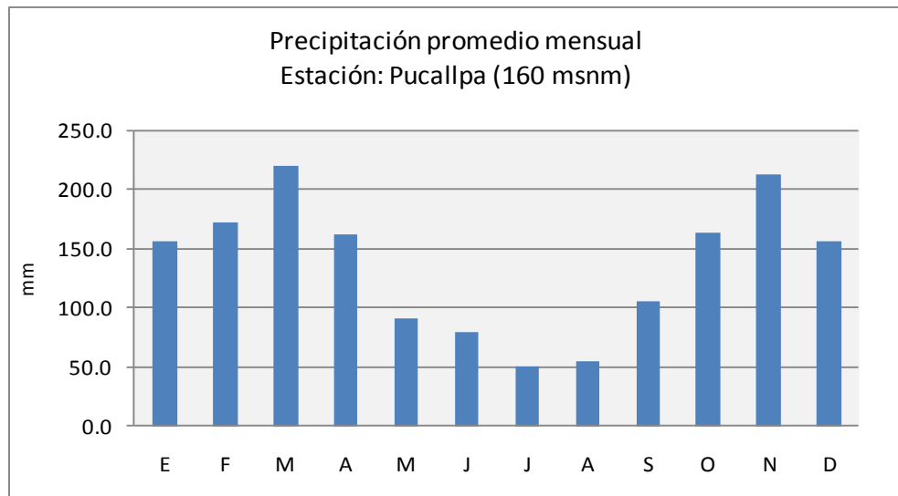
Figura 2. Ciclo anual de la precipitación en la estación Pucallpa (160 msnm).
