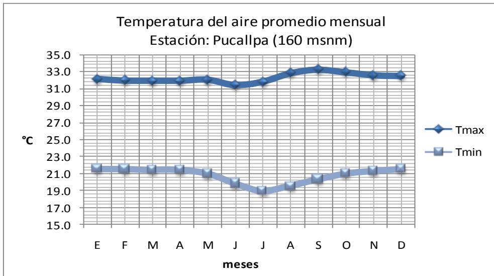
Figura 1. Ciclo anual de las temperaturas extremas del aire en la estación Pucallpa (160 msnm).
