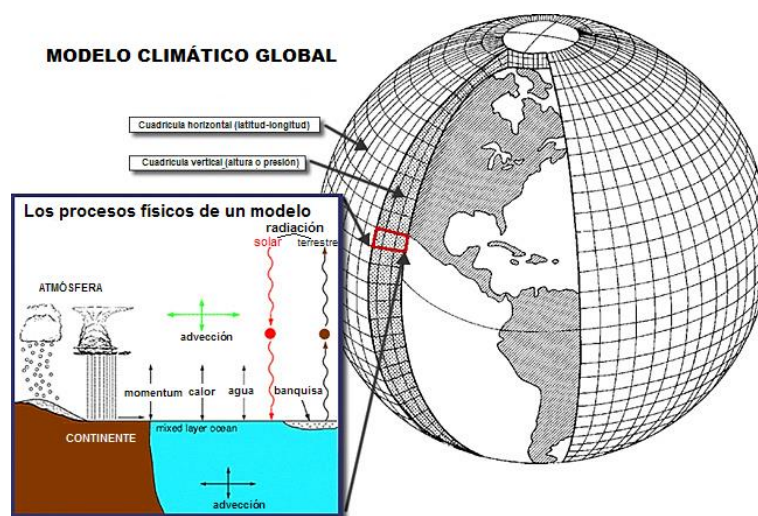
Figura 3. Esquema de un modelo climático global. Fuente NOAA
