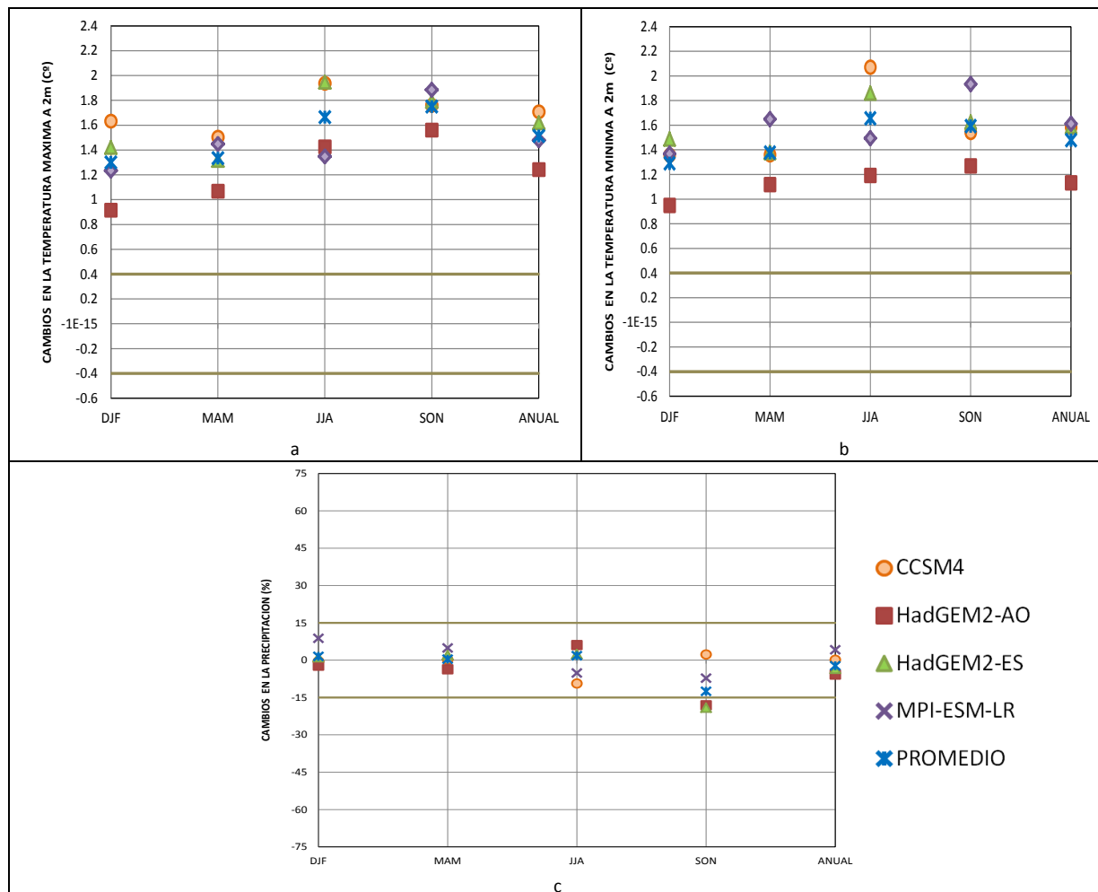
Figura 7. Cambios proyectados a nivel anual y estacional (DEF-verano; MAM-otoño; JJA-invierno; SON-primavera) de la temperatura del aire máxima (a), mínima (b) en °C, y de la precipitación (c) en porcentajes en la Región Ucayali para el time-slice centrado en el año 2030, relativo al período de referencia 1971-2000. Los modelos son: CCSM4, HadGEM2-AO, HadGEM2-ES y MPI-ESM-LR, para el escenario de emisiones RCP8.5. Se muestra el promedio de los modelos (X azul) y los rangos de la variabilidad actual (líneas verdes horizontales).
