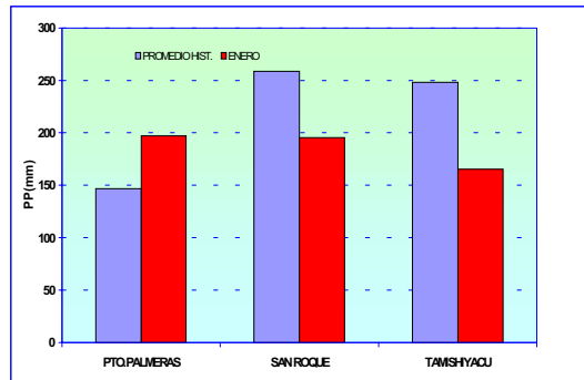
Gráfico 22. Histograma de precipitaciones en la sub cuenca Amazonas
