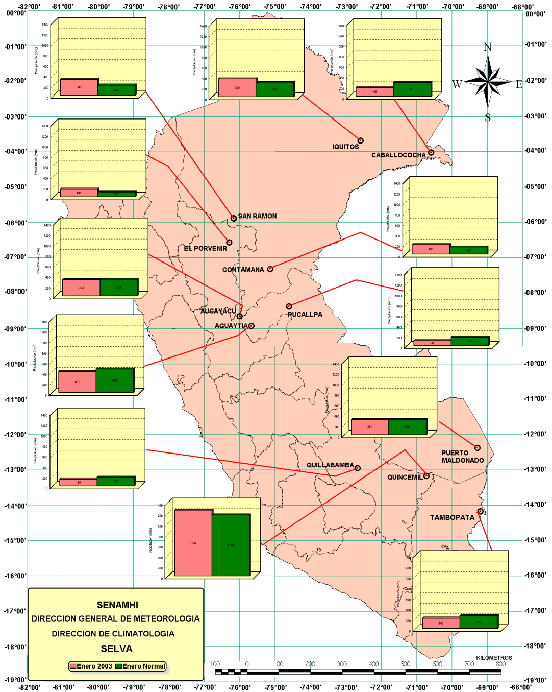
Mapa 4. Lluvias acumuladas en la selva en lo que va del periodo lluvioso 2002/2003
