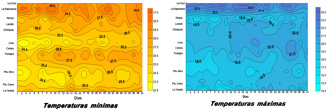
Figura 14. Temperatura extremas del aire en estaciones costeras ( °C )
