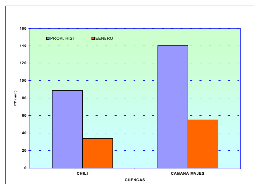
Figura 9 .Histograma de precipitación media zona sur de la vertiente del océano Pacífico
