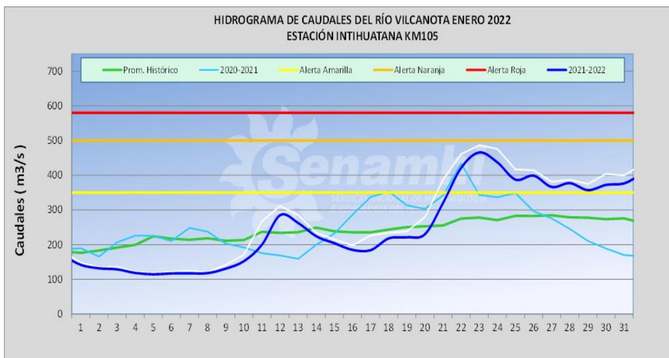
Figura 10. Hidrograma estación Intihutana km 105 mes de enero del 2022
