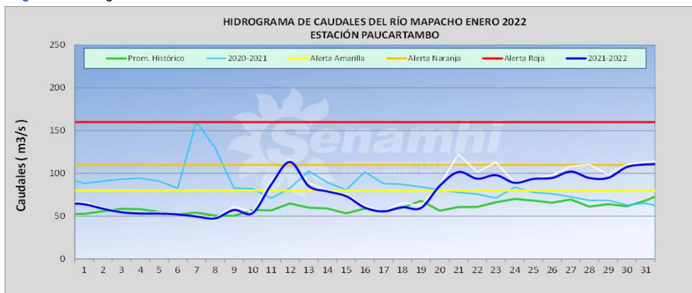
Figura 12. Hidrograma estación Paucartambo mes de enero del 2022
