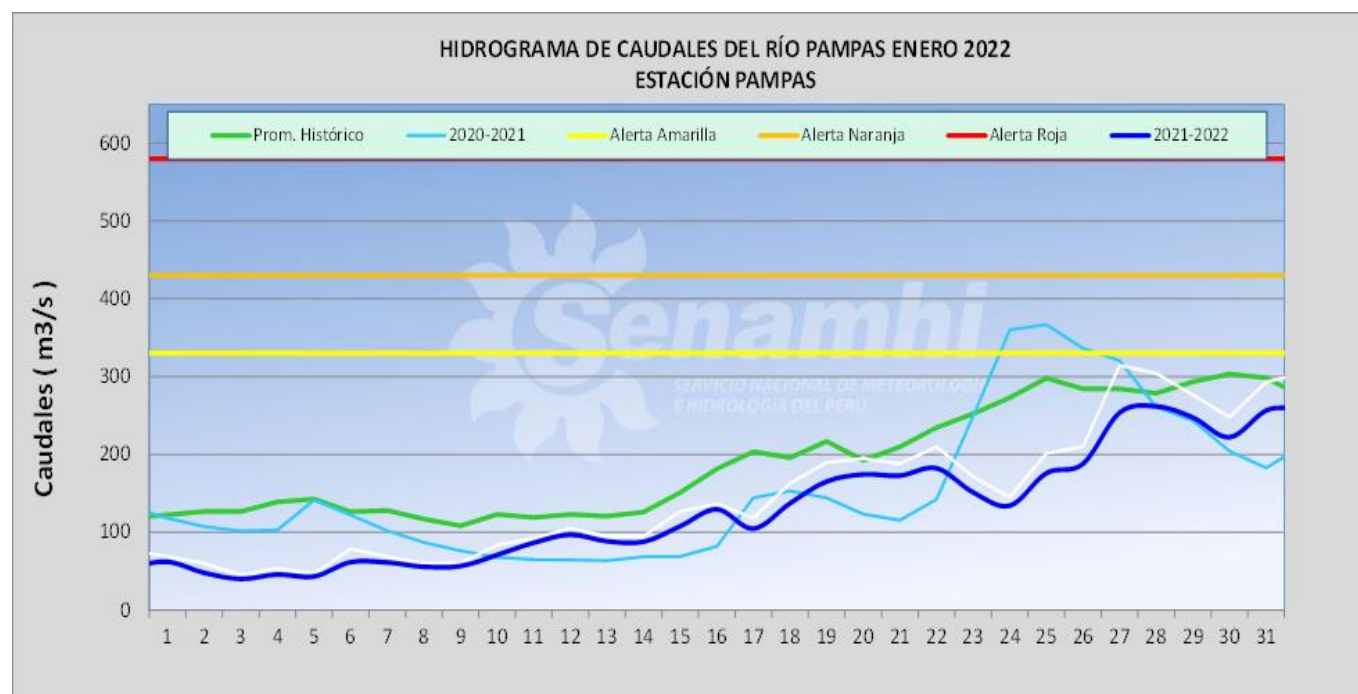
Figura 17. Hidrograma estación Puente Pampas mes de enero del 2022
