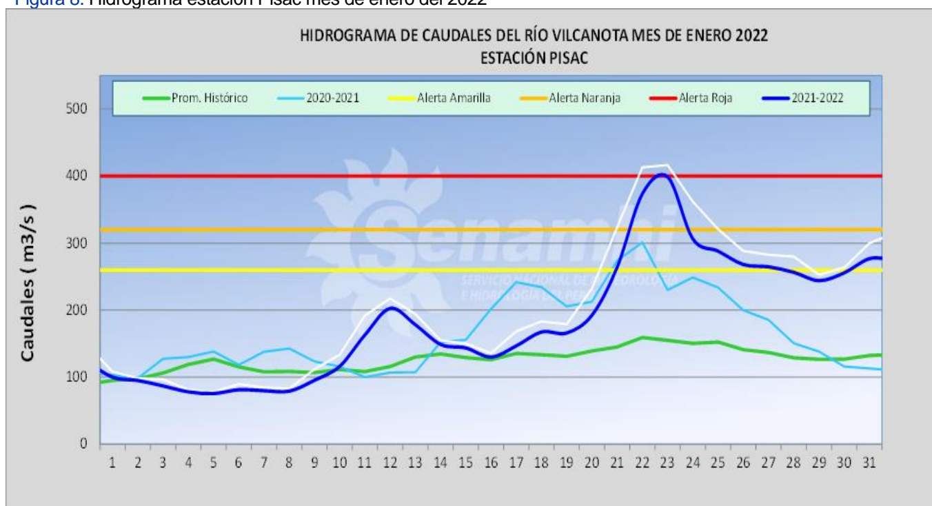
Figura 8. Hidrograma estación Pisac mes de enero del 2022
