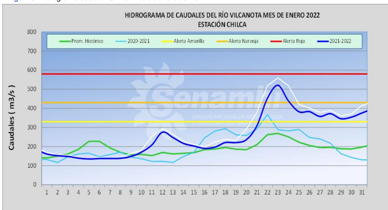
Figura 9. Hidrograma estación Chilca mes de enero del 2022
