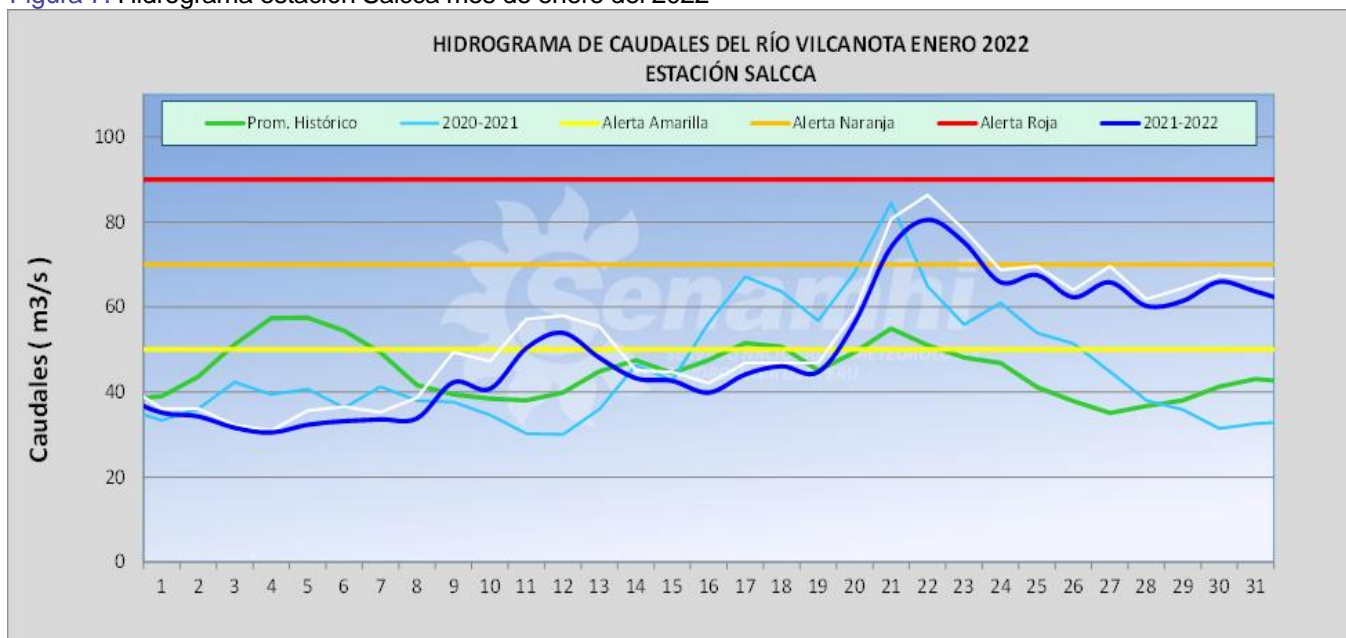
Figura 7. Hidrograma estación Salcca mes de enero del 2022
