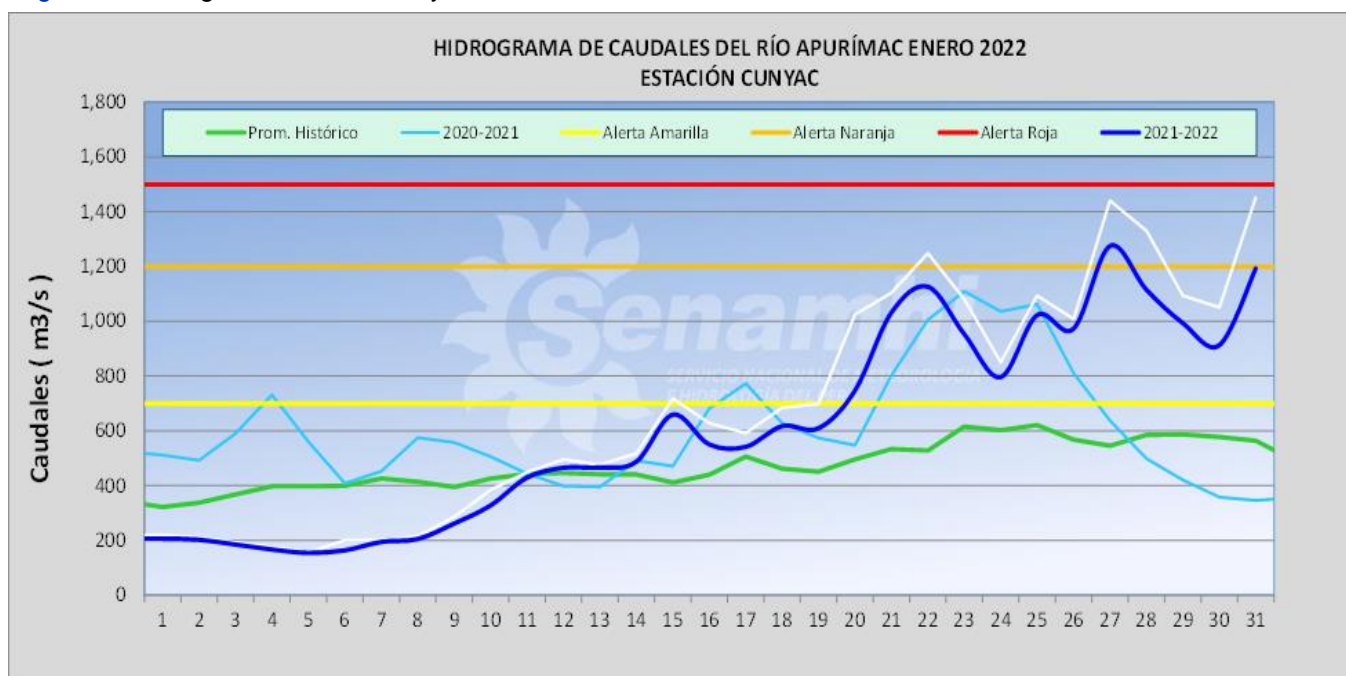
Figura 14. Hidrograma estación Cunyac mes de enero del 2022
