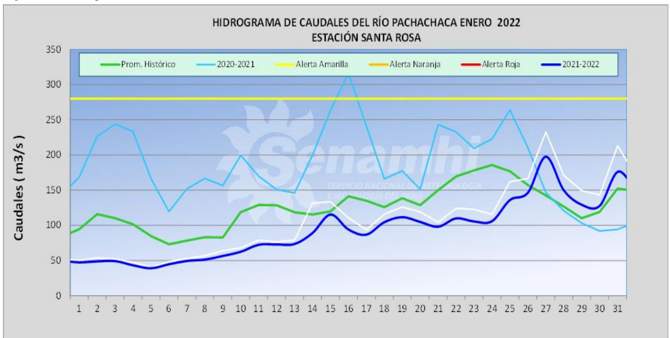
Figura 15. Hidrograma estación Santa Rosa mes de enero del 2022
