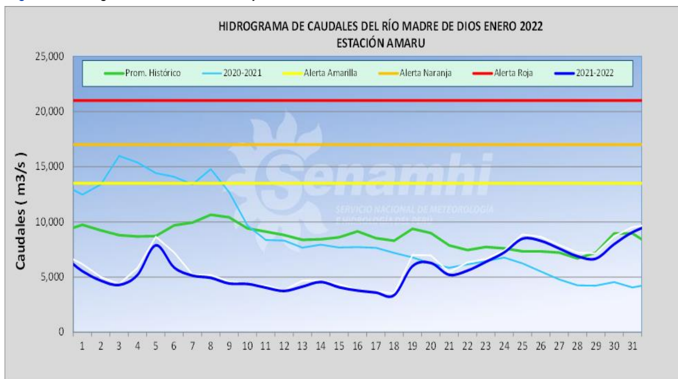
Figura 19. Hidrograma estación Amaru Mayo mes de enero del 2022
