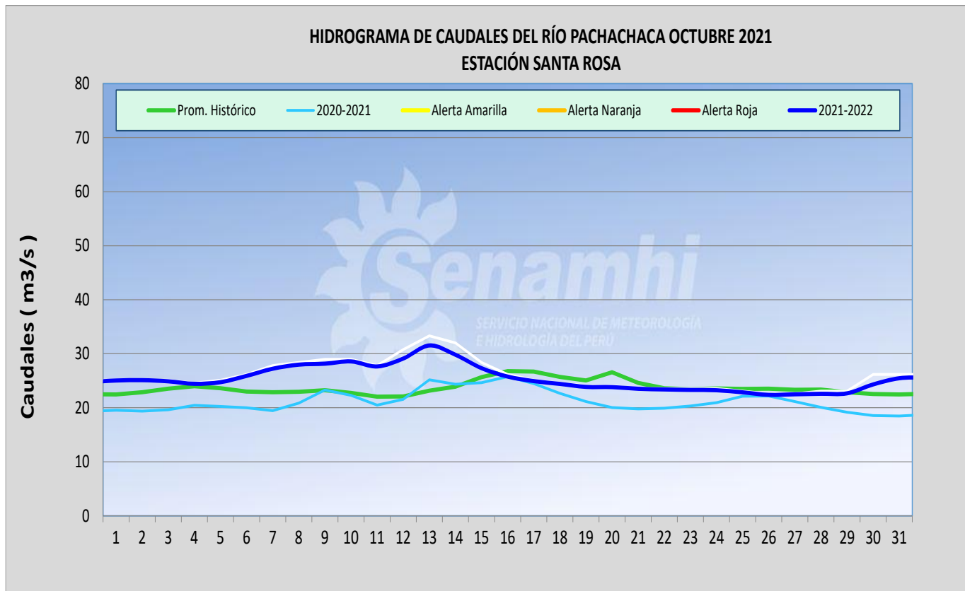
Figura 15. Hidrograma estación Santa Rosa mes de octubre del 2021
