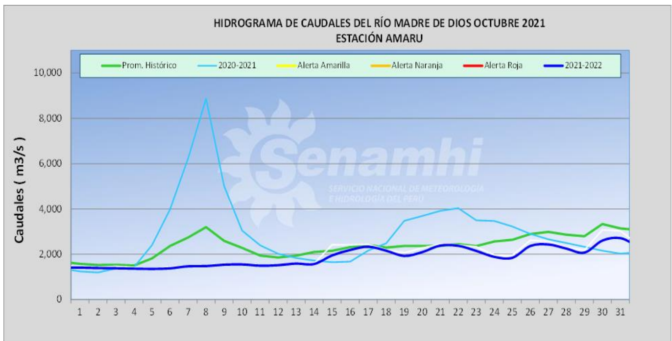
Figura 19. Hidrograma estación Amaru Mayo mes de octubre del 2021
