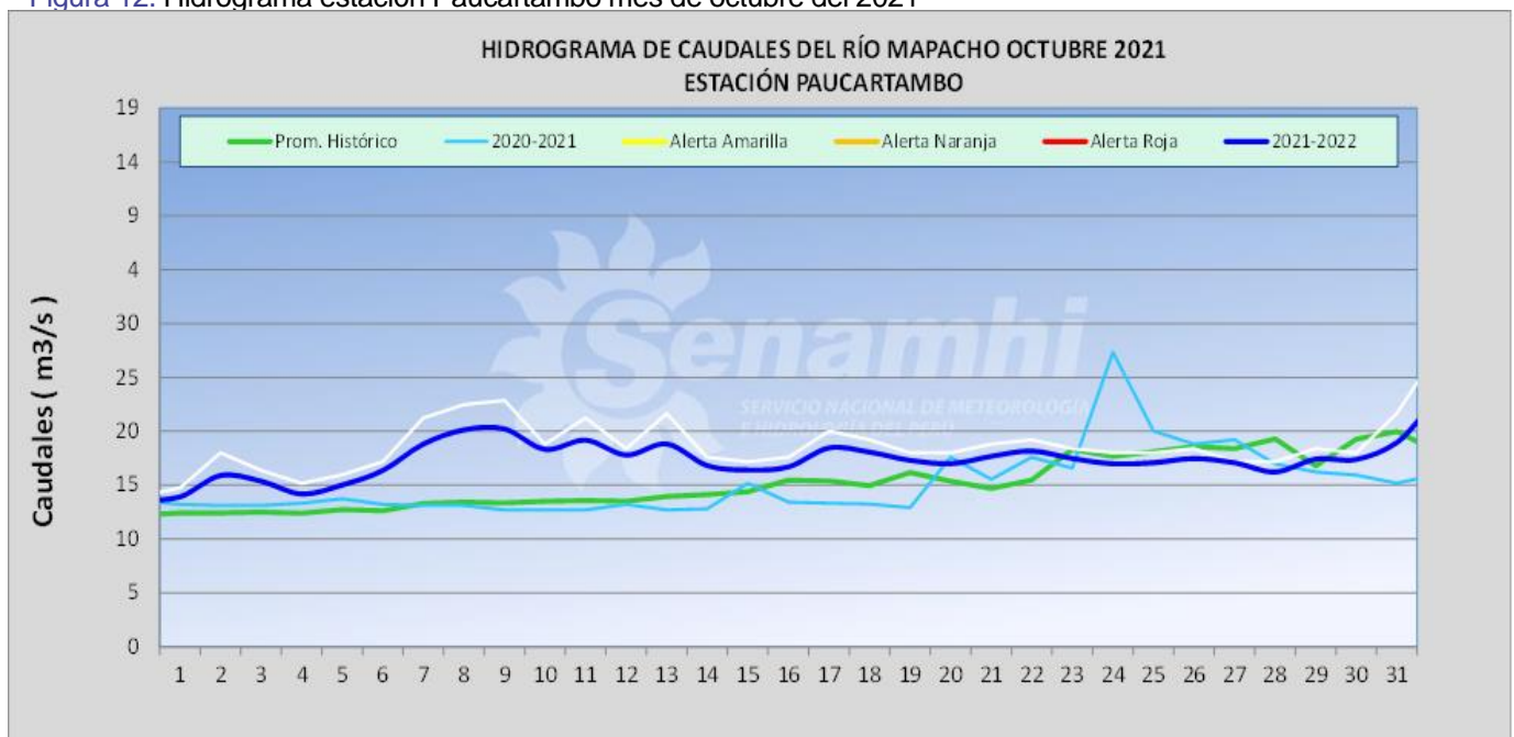
Figura 12. Hidrograma estación Paucartambo mes de octubre del 2021
