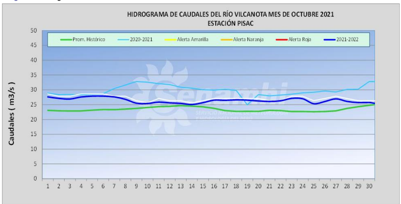
Figura 8. Hidrograma estación Pisac mes de octubre del 2021
