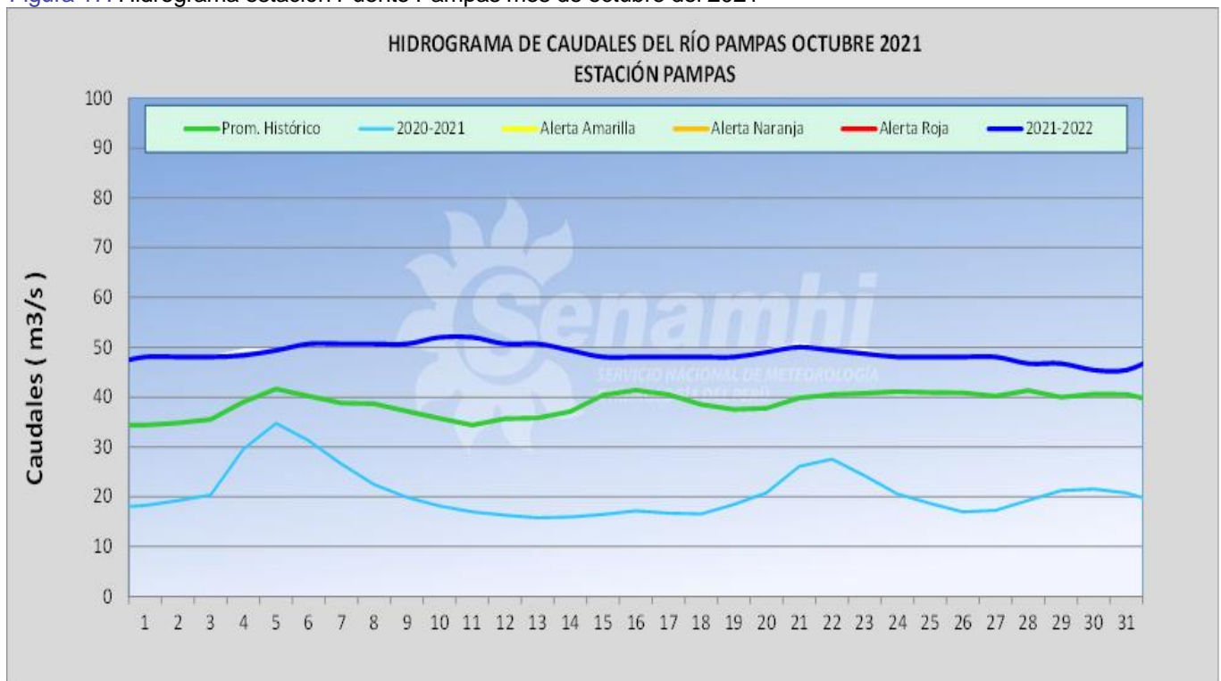
Figura 17. Hidrograma estación Puentes Pampas mes de octubre del 2021
