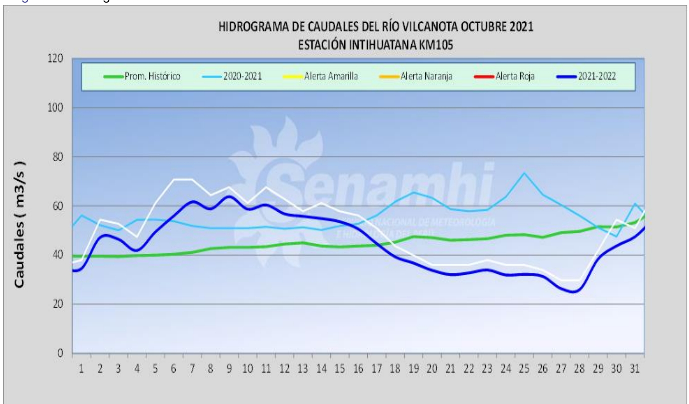
Figura 10. Hidrograma estación Intihutana km 105 mes de octubre del 2021
