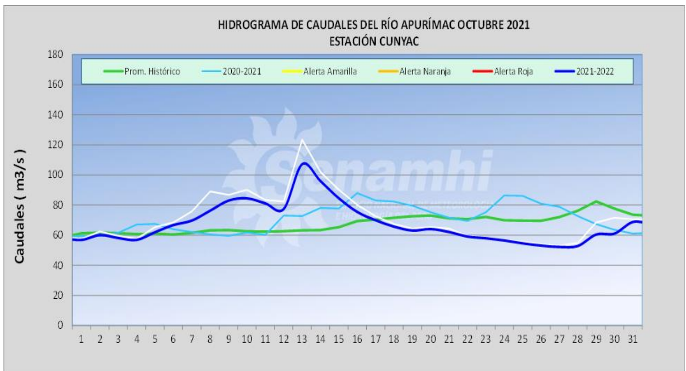
Figura 14. Hidrograma estación Cunyac mes de octubre del 2021
