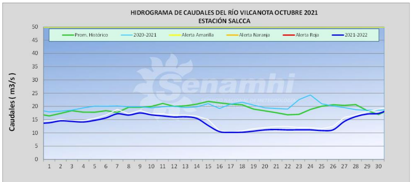
Figura 7. Hidrograma estación Salcca mes de octubre del 2021
