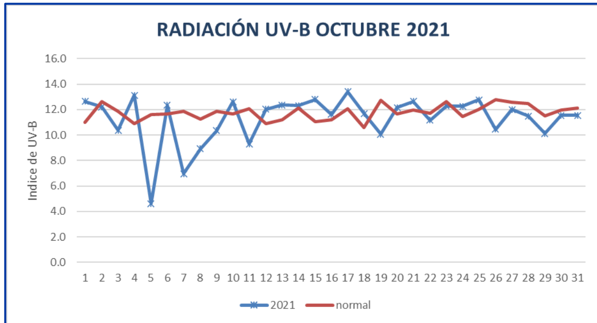
Figura 21. Radiación diaria UV-B octubre 2021.
