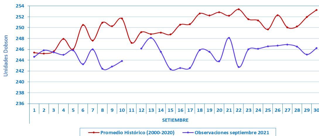
Comportamiento temporal de la concentración de ozono atmosférico en la Estación VAG Marcapomacocha. Setiembre 2021.
