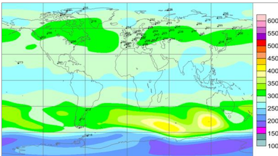
Mapa de ozono total atmosférico para el mes de setiembre 2021
