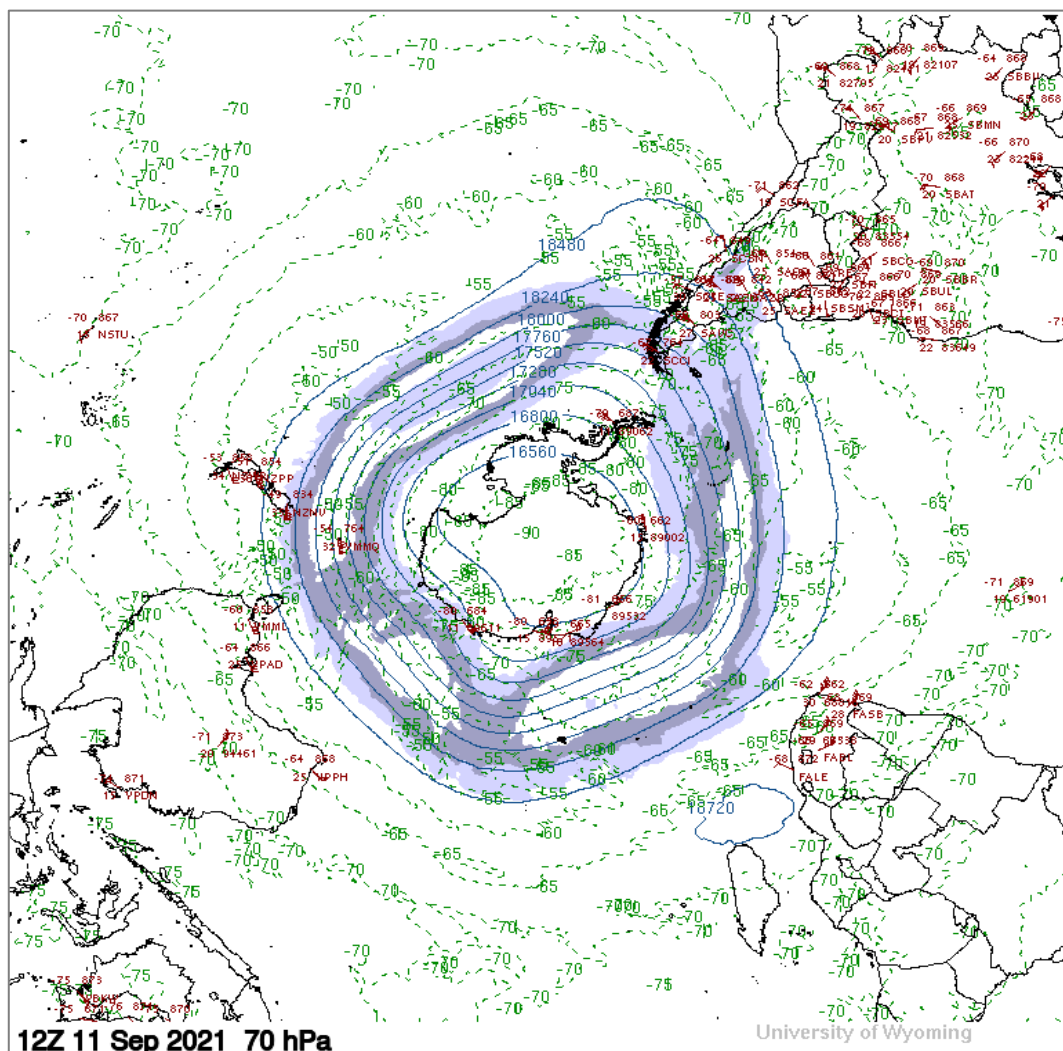
Comportamiento de la temperatura en 70 hPa para el hemisferio sur (11 setiembre 2021)
