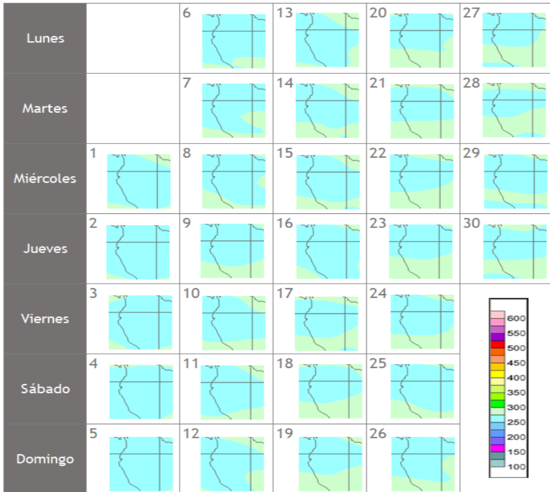
Mapa diario del ozono total atmosférico para el mes de setiembre 2021.
