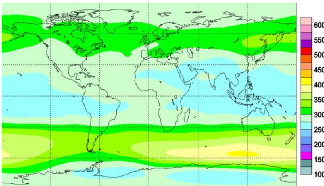
Mapa Climático de ozono total atmosférico (1978 – 1988) para el mes de setiembre.
