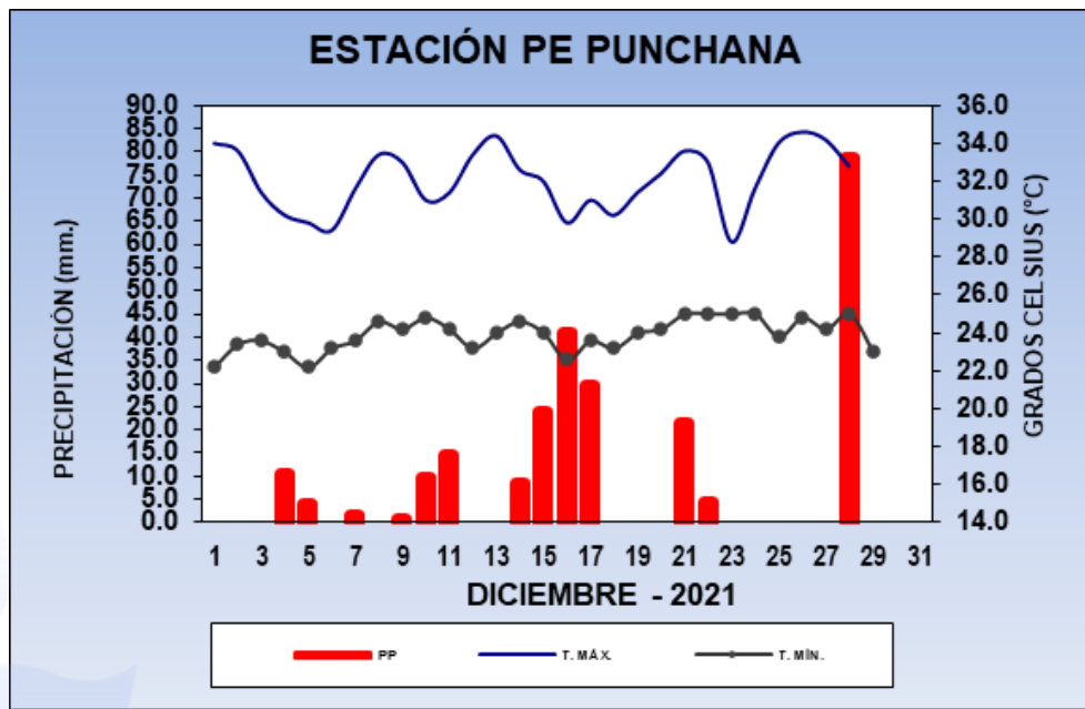
Gráfico N° 02: Registro termopluviométrico de la estación Punchana – Diciembre 2021.
