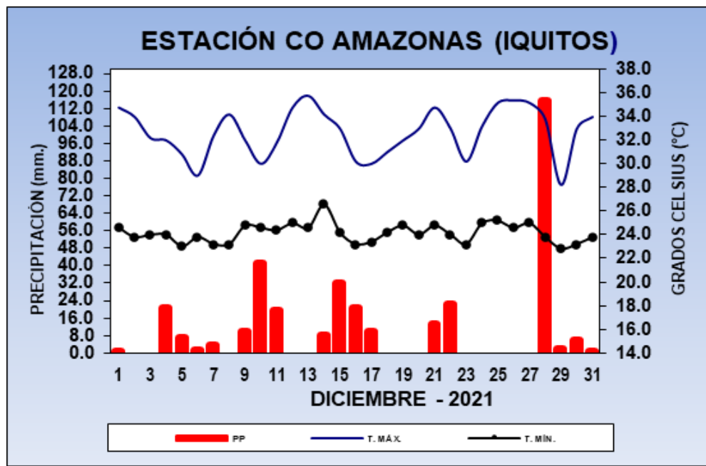
Gráfico N° 06: Registro termoplumiométrico de la estación Amazonas Iquitos – Diciembre 2021.
