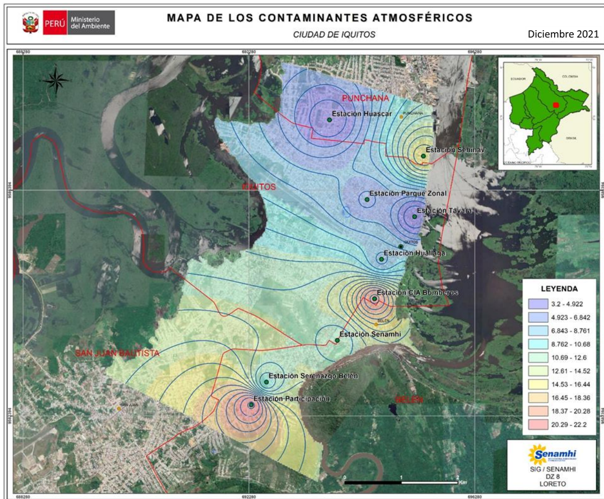
Mapa N° 04: Contaminantes atmosféricos en la ciudad de Iquitos, correspondiente al mes de diciembre 2021.
