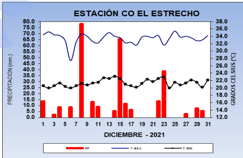
Gráfico N° 03: Registro termopluviométrico de la estación El Estrecho – Diciembre 2021.
