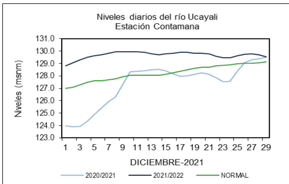
Gráfico N° 13: Niveles diarios del río Uçayali (Estación Contamana).
