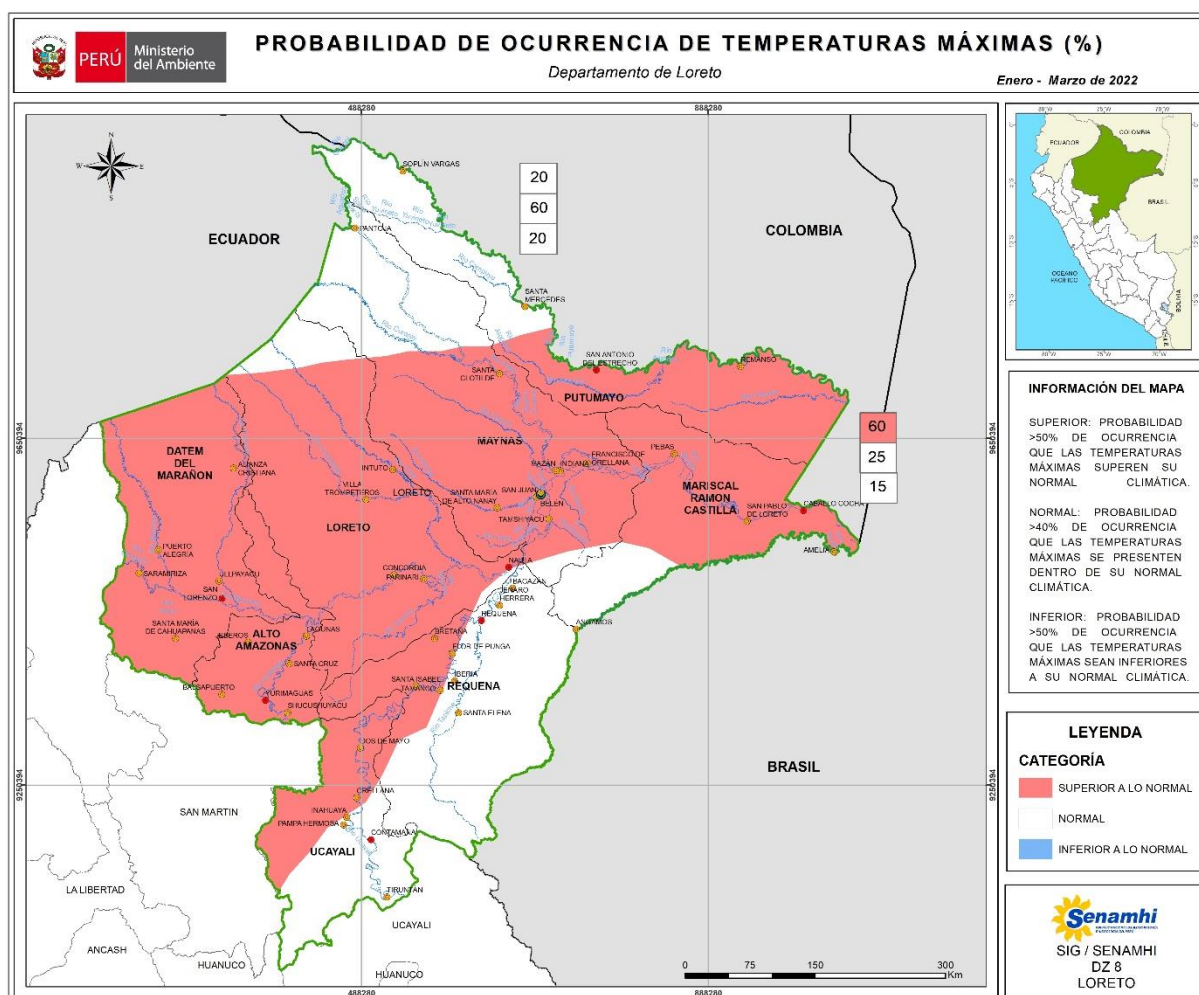
Mapa N° 02: Probabilidad de ocurrencia de temperatura máxima del mes de enero a marzo de 2022.
