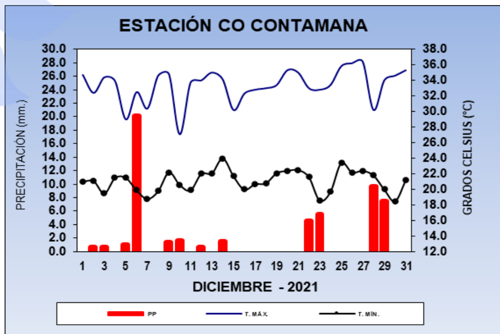
Gráfico N° 05: Registro termopluviométrico de la estación Contamana – Diciembre 2021.
