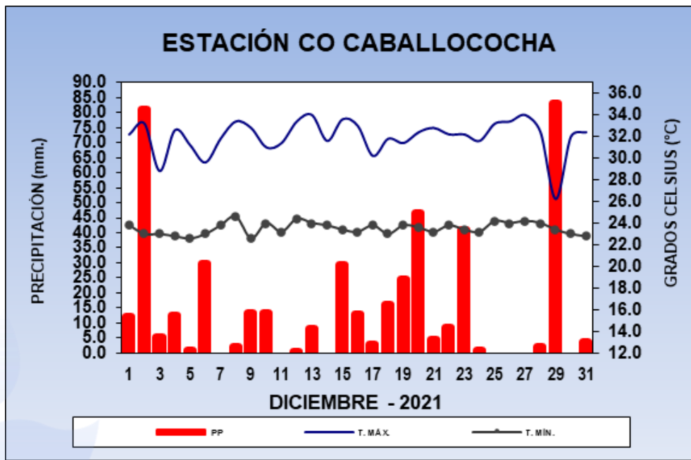
Gráfico N° 04: Registro termopluviométrico de la estación Caballococha – Diciembre 2021.
