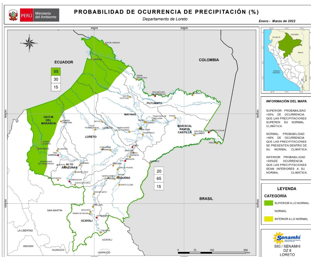
Mapa N° 01: Probabilidad de ocurrencia de precipitación del mes de enero a marzo de 2022.
