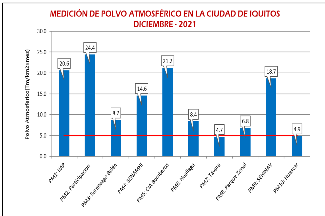
Gráfico N° 18: Medición de polvo atmosférico en la ciudad de Iquitos, correspondiente al mes de Diciembre 2021.
