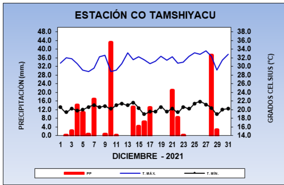
Gráfico N° 01: Registro termopluviométrico de la estación Tamshiyacu – Diciembre 2021.
