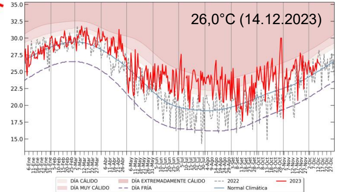
TEMPERATURA MÁXIMA [°C] ESTACIÓN: VON HUMBOLDT - LIMA
