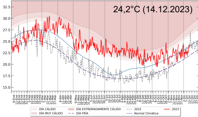
TEMPERATURA MÁXIMA [°C] ESTACIÓN: AEROPUERTO INTERNACIONAL - CALLAO
