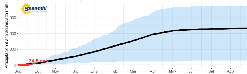
PRECIPITACIÓN DIARIA ACUMULADA DE SEPTIEMBRE A AGOSTO - ESTACIÓN CERRO_DE_PASCO
