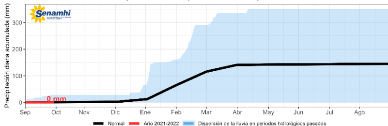
PRECIPITACIÓN DIARIA ACUMULADA DE SEPTIEMBRE A AGOSTO - ESTACIÓN SITAJARA
