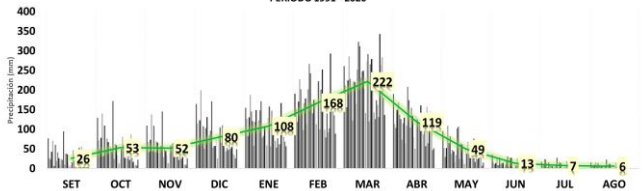
SIERRA NORTE OCCIDENTAL PERIODO 1991 - 2020
