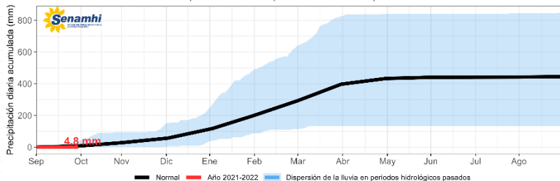
PRECIPITACIÓN DIARIA ACUMULADA DE SEPTIEMBRE A AGOSTO - ESTACIÓN SHEQUE
