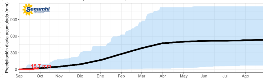
PRECIPITACIÓN DIARIA ACUMULADA DE SEPTIEMBRE A AGOSTO - ESTACIÓN CAY_CAY
