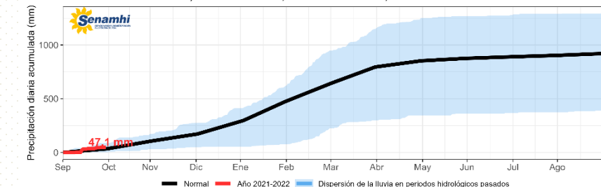
PRECIPITACIÓN DIARIA ACUMULADA DE SEPTIEMBRE A AGOSTO - ESTACIÓN COLCABAMBA
