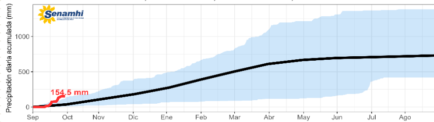
PRECIPITACIÓN DIARIA ACUMULADA DE SEPTIEMBRE A AGOSTO - ESTACIÓN COLCABAMBA
