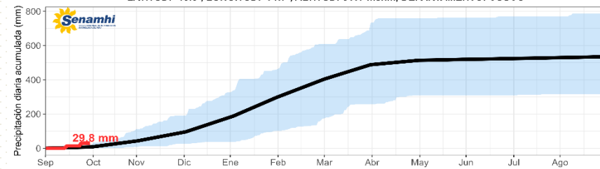
PRECIPITACIÓN DIARIA ACUMULADA DE SEPTIEMBRE A AGOSTO - ESTACIÓN DESAGUADERO
