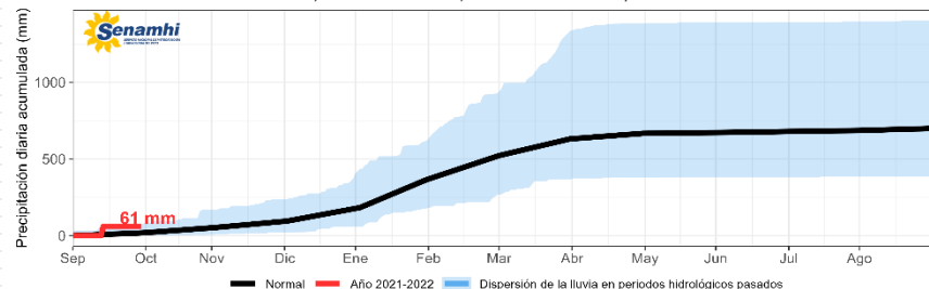
PRECIPITACIÓN DIARIA ACUMULADA DE SEPTIEMBRE A AGOSTO - ESTACIÓN DESAGUADERO
