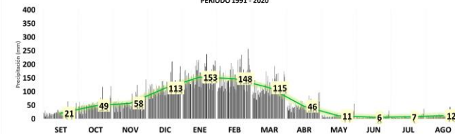
SIERRA SUR ORIENTAL PERIODO 1991 - 2020
