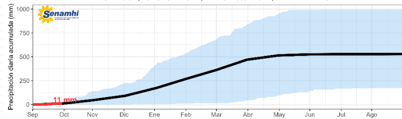
PRECIPITACIÓN DIARIA ACUMULADA DE SEPTIEMBRE A AGOSTO - ESTACIÓN SHEQUE
