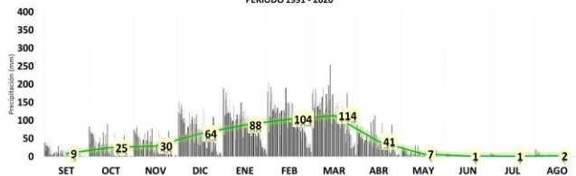
SIERRA CENTRAL OCCIDENTAL PERIODO 1991 - 2020
