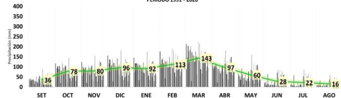
SIERRA NORTE ORIENTAL PERIODO 1991 - 2020
