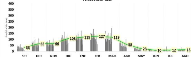
SIERRA CENTRAL ORIENTAL PERIODO 1991 - 2020
