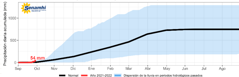
PRECIPITACIÓN DIARIA ACUMULADA DE SEPTIEMBRE A AGOSTO - ESTACIÓN YUNGAY
