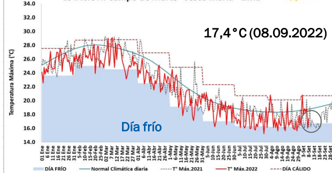
TEMPERATURA MÁXIMA : ENERO - SETIEMBRE 2022 ESTACIÓN: Campo de Marte - Jesús María - Lima
