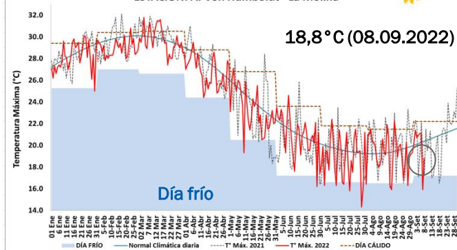
TEMPERATURA MÁXIMA : ENERO - SETIEMBRE 2022 ESTACIÓN: A. Von Humboldt - La Molina
