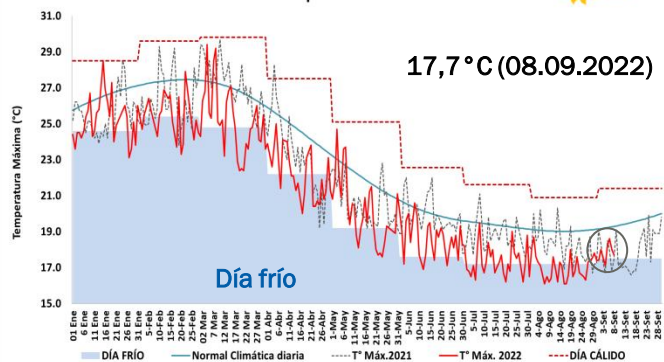
TEMPERATURA MÁXIMA : ENERO - SETIEMBRE 2022 ESTACIÓN: Aeropuerto Internacional - Callao
