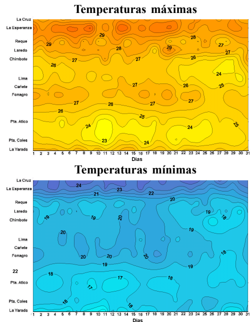
Figura 11. Temperaturas extremas del aire en estaciones costeras
