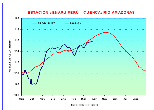
Gráfico 19. Limnigrama de niveles diarios del río Amazonas
