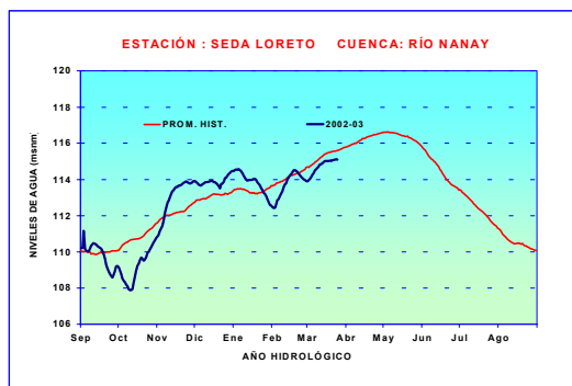
Gráfico 20. Limnigrama de niveles diarios del río Nanay
