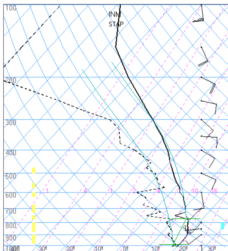
Figura 6. Radiosondaje mensual promedio - marzo 2003 (Aeropuerto Internacional Jorge Chávez)
