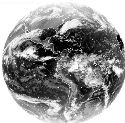
Figura 6. Imagen de Satélite - GOES 8 para el día 24 de marzo de 2003 a las 12:00 UTC
