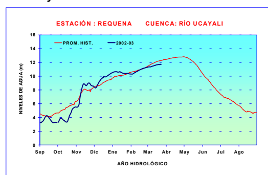
Gráfico 23. Limnigrama de niveles diarios del río Ucayali
